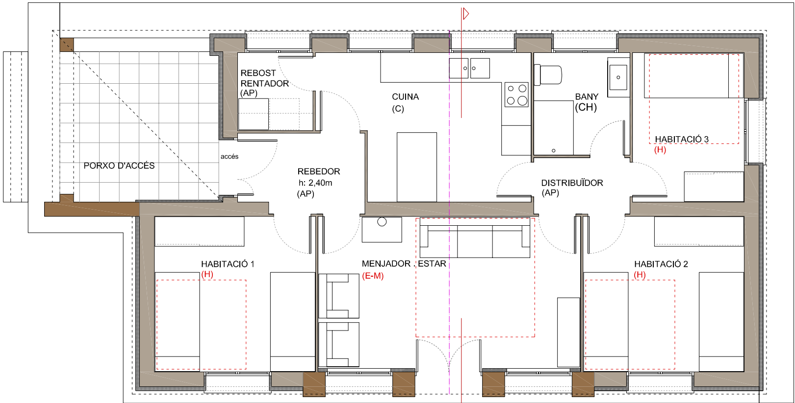
PLANTA DE DISTRIBUCIÓ DE L'HABITATGE
