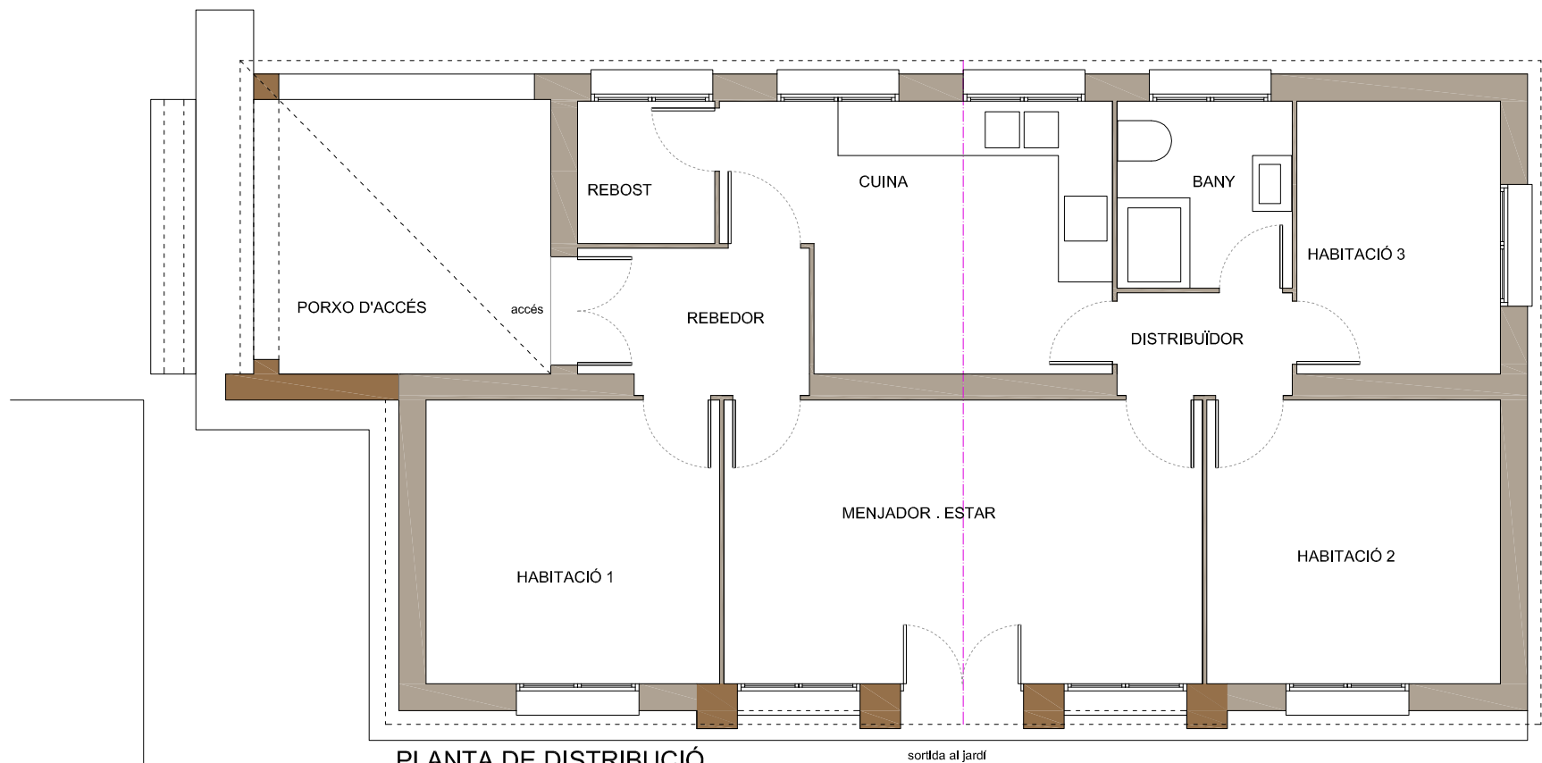
PLANTA DE DISTRIBUCIÓ
