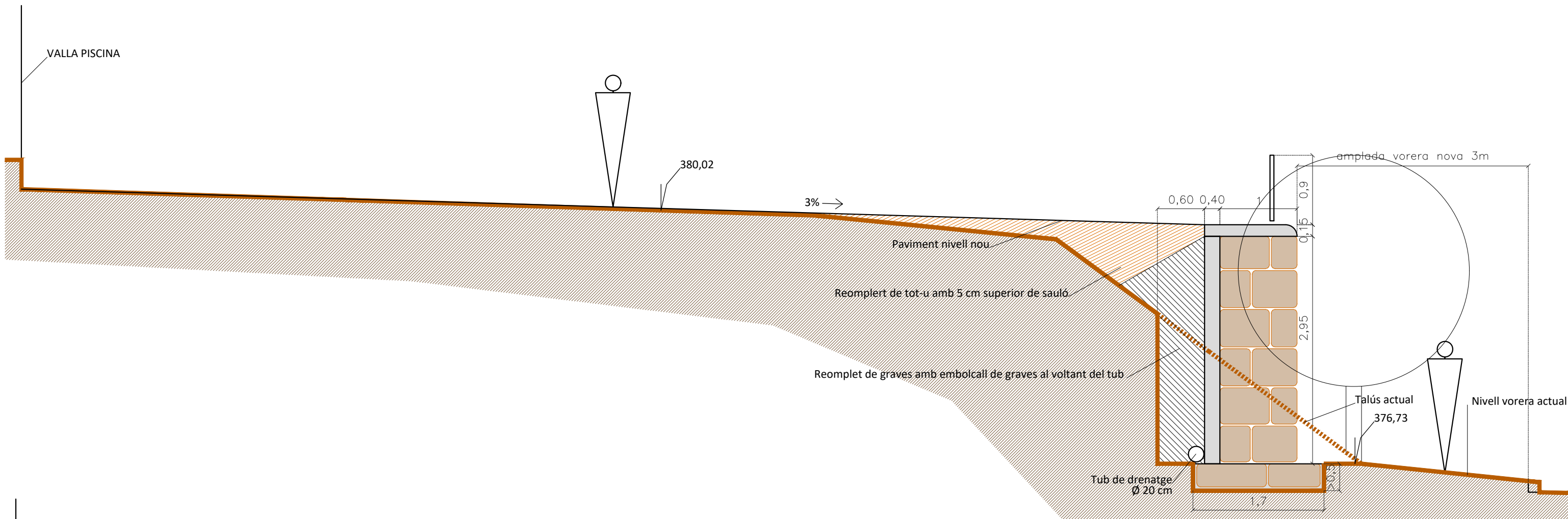
SECCIÓ TRANSVERSAL 3
