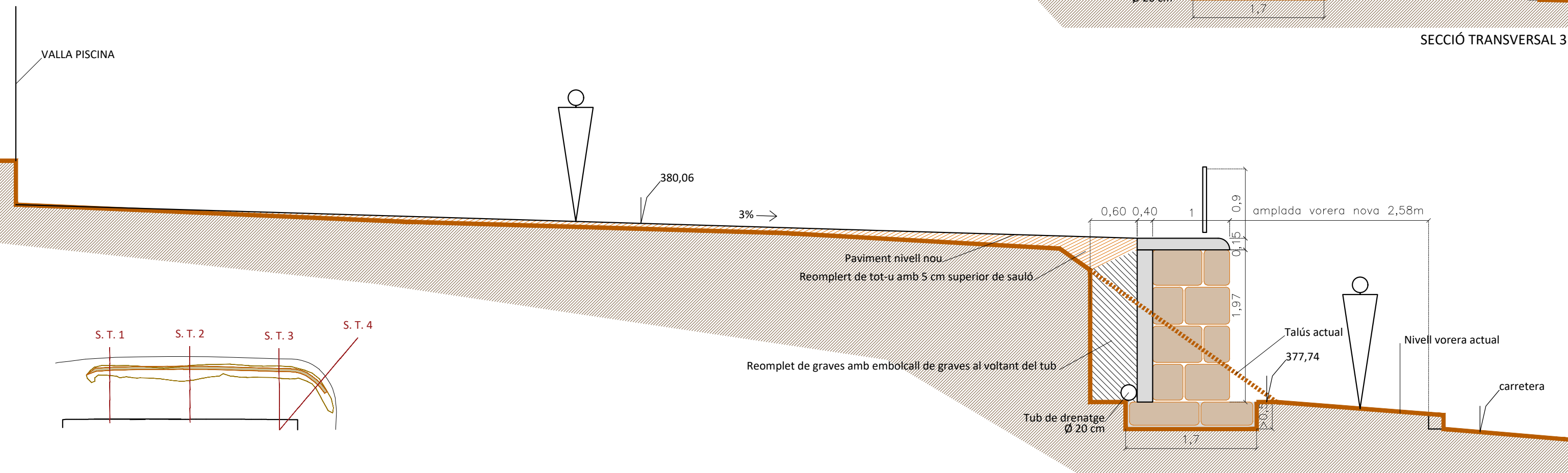
SECCIÓ TRANSVERSAL 4
