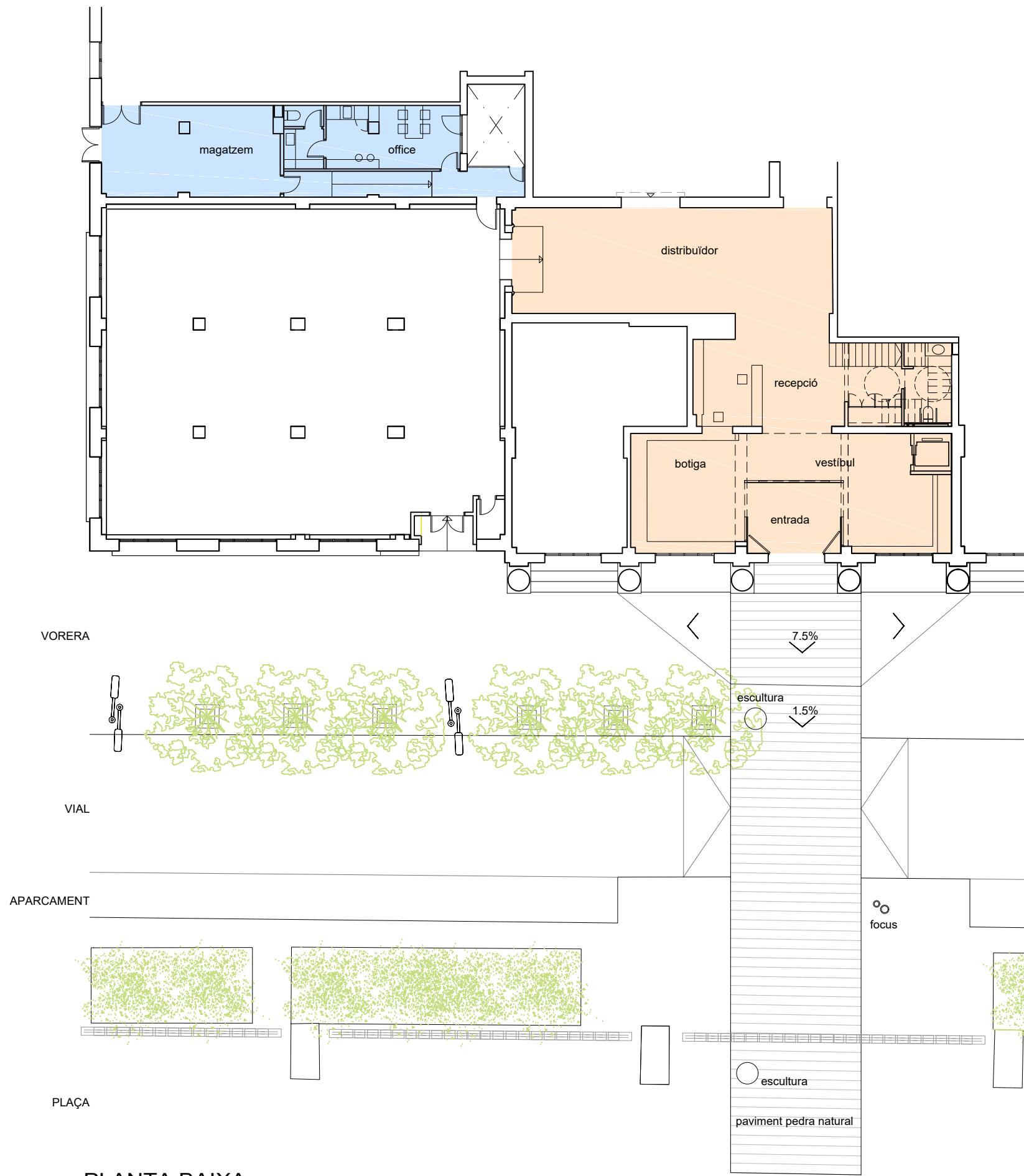
PLANTA BAIXA
