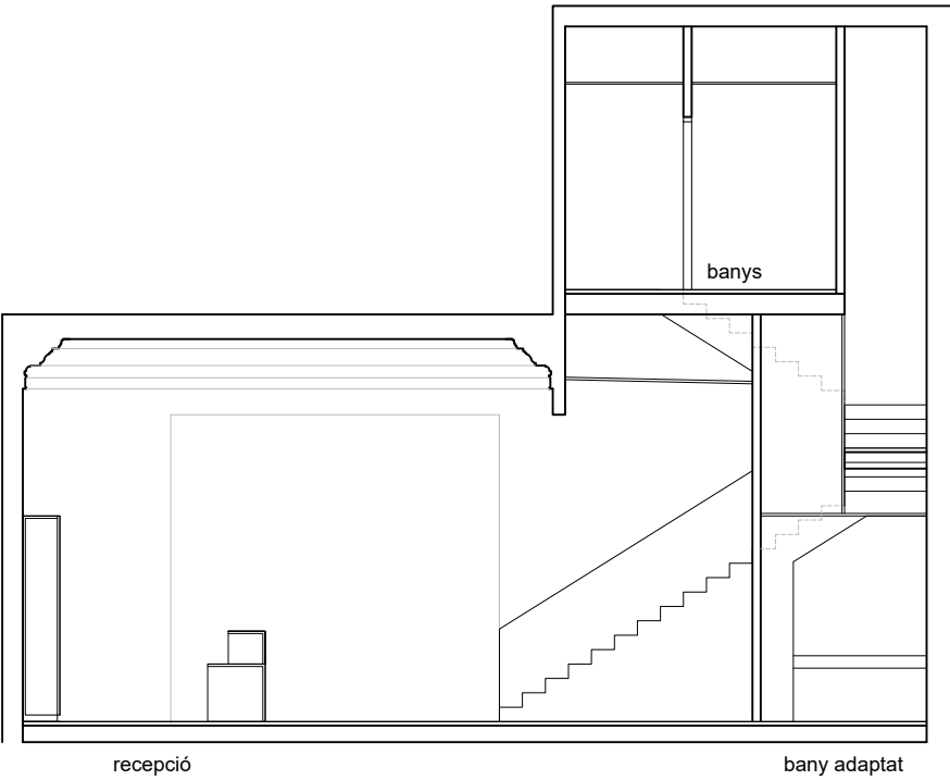
SECCIÓ 2
