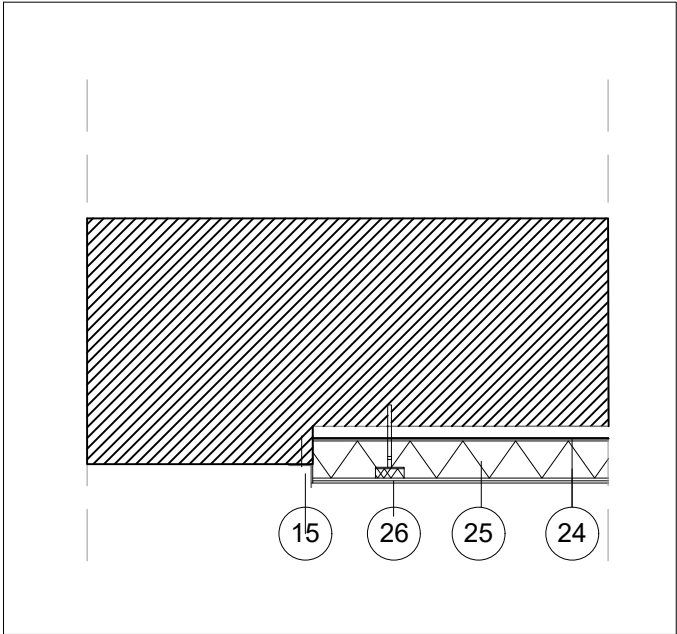
DETALL F (ENTREGA SATE AMB AGULLA OBRA VISTA)
