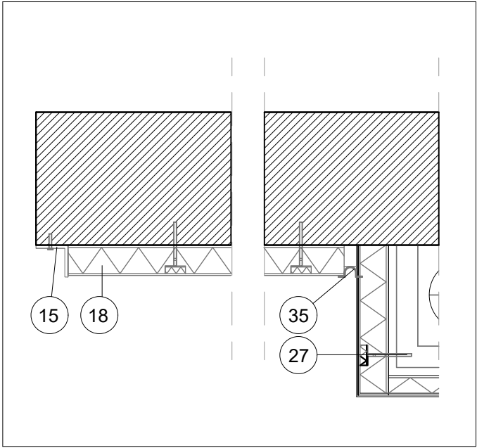
DETALL A (FAÇANA-RÂFEC)
