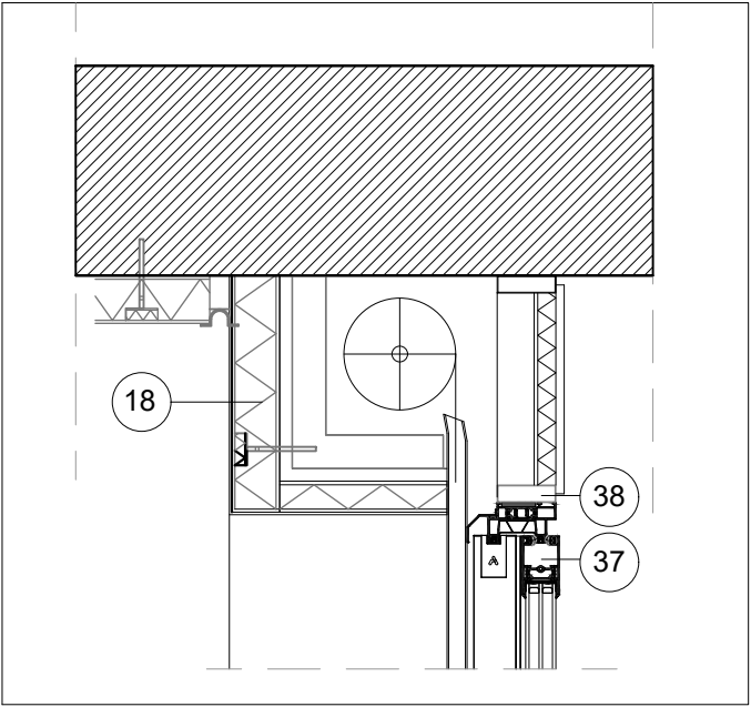
DETALL B (DINTELL)
