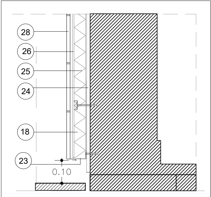
DETALL D (SÒCOL CERÀMIC)
