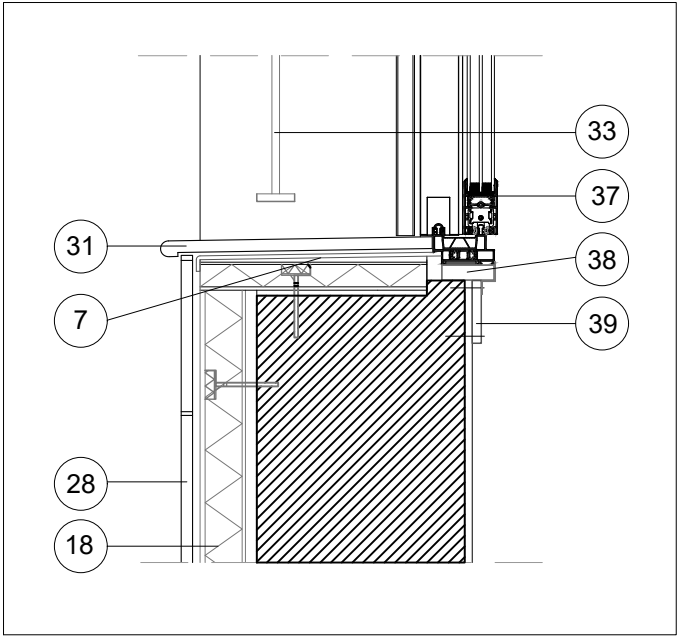
DETALL C (AMPIT)
