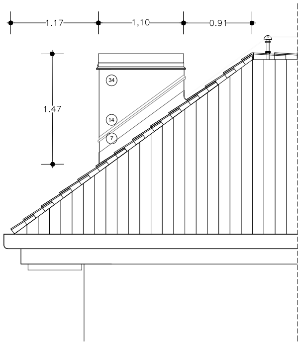
DETALL SORTIDA COBERTA 1/50
