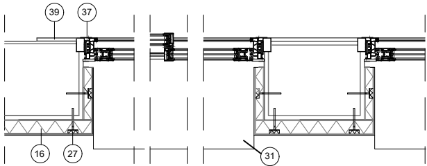
PLANTA REFORMADA (NIVELL FINESTRES)
