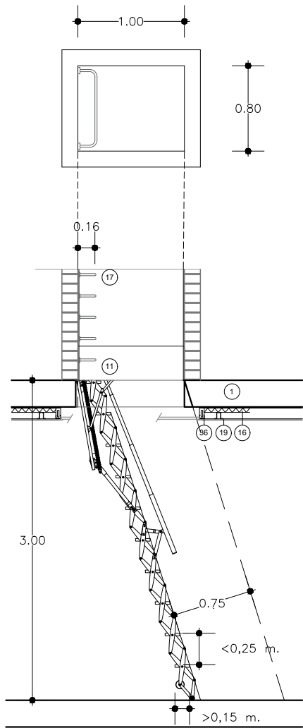
SECCIÓ PER ESCALA ESCAMOTEJABLE 1/50 (MIDES A REPLANTEJAR EN OBRA)
