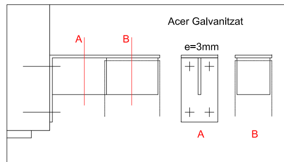
DETALL ANCORATGE MUNTANT LAMES
