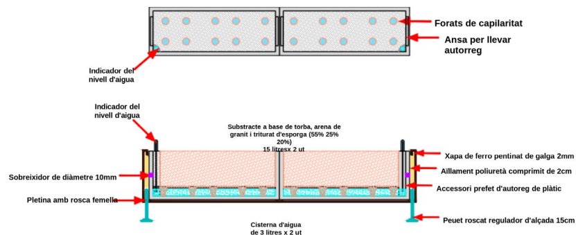
Jardinera ferro pentinat 1040x230x200 amb 2mm de galga
