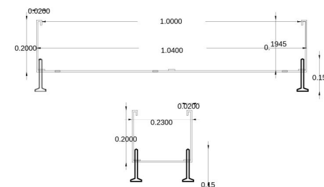
Secció frontal jardinera 1040x230x200
