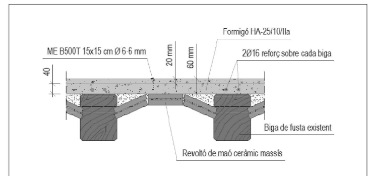
DETALL 1: Reforç del 2n sostre
