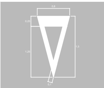
E-74c Cediu el pas en un carril bicicleta
