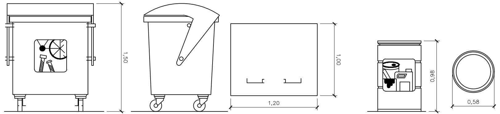
CONTENIDOR DE 1000L. APTE PER A PAPER I CARTRÓ, PLÀSTICS.
