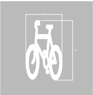
E-77 Bicicleta Es col·locarà en els carrils bicicleta Amplada Carril (L) Amplada Logo (A) 80 < L < 100 80 100 < L < 120 95 120 < L < 160 110 L > 160 150 ACTUALITZAT 2017
