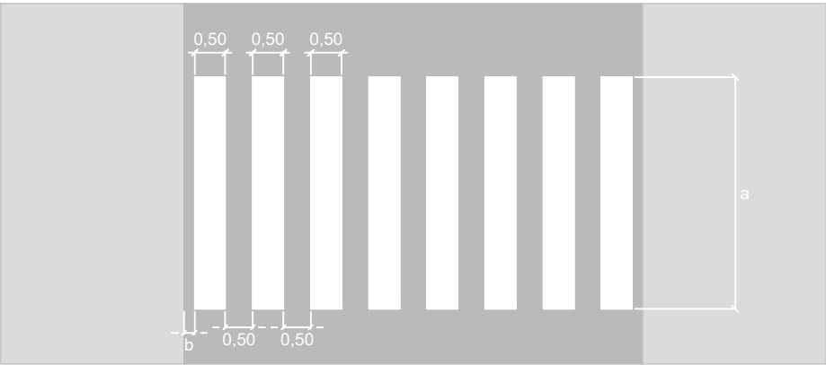
E-4a Pas de vianants sense semàfors L'amplada a del pas de vianants serà com a mínim de 4 m, i com a norma general de 5 m. En calçades de poca amplada i amb velocitats no superiors a 40 km/h, el valor de a pot reduir-se a 2,5 m. Les dues bandes més properes a la vora de la calçada o de la vorada han d'estar a una distància b, entre 0 i 0,50 cm. En una via de doble sentit de circulació, es procurarà que l'eix de la marca de separació dels sentits coincideixi amb l'eix d'una banda del pas o amb l'eix d'una interbanda.
