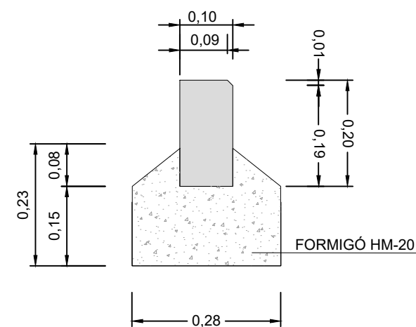
DETALL VORADA RECTA TIPUS FIOL - V05 - E:1/10
