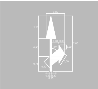
E-43 Recta a la dreta (a l'esquerra) La flexa de direcció a l'esquerra és la simètrica respecte a un eix longitudinal.
