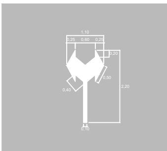
E-44 A la dreta o a l'esquerra
