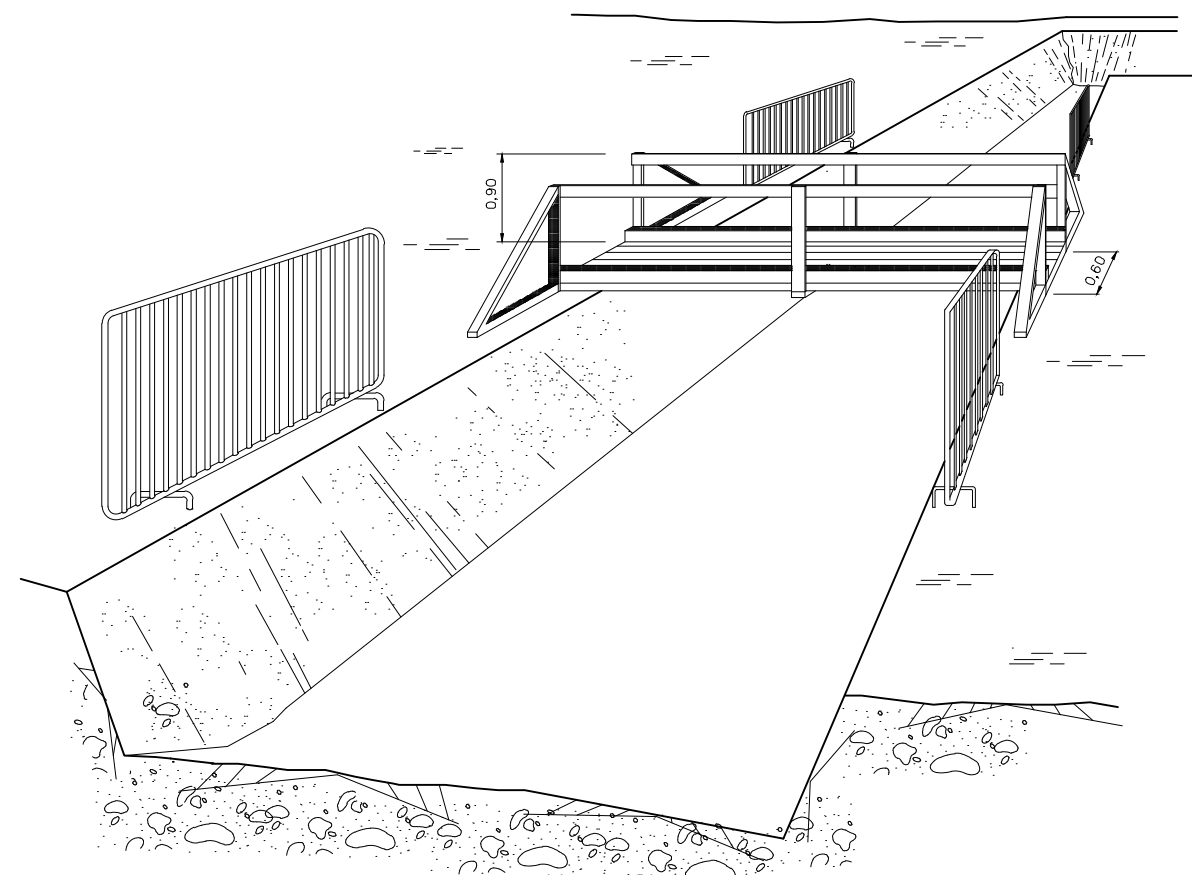
PASSOS SOBRE RASES
