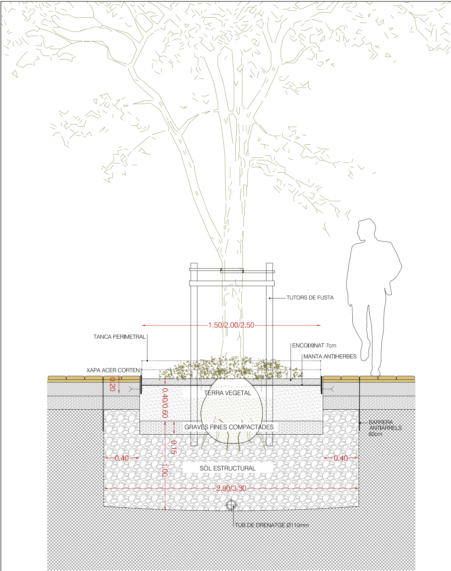
DETALL ESCOCELL Sòl estructural (composició per m3): 1 M3 de graves d'arestes vives de granulometria 4-6 cm sense fins i 0.2 m3 de terra vegetal
