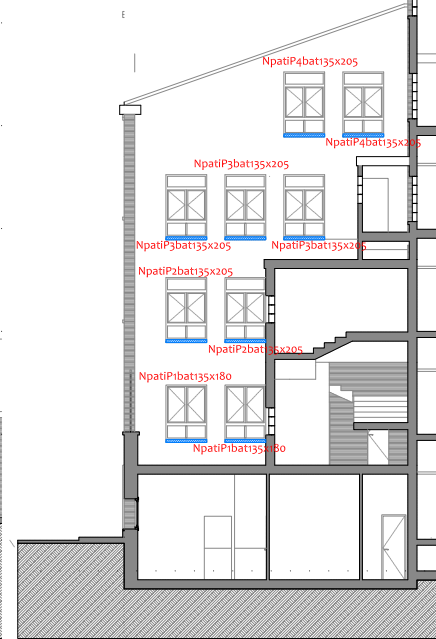
SECCIÓ E-E'
