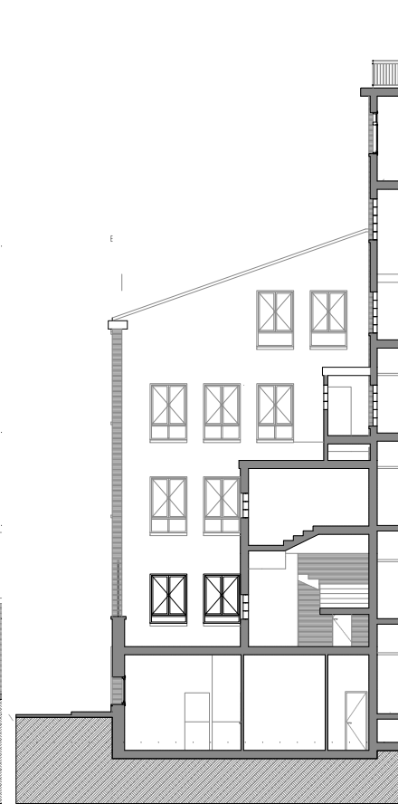
SECCIÓ E-E'
