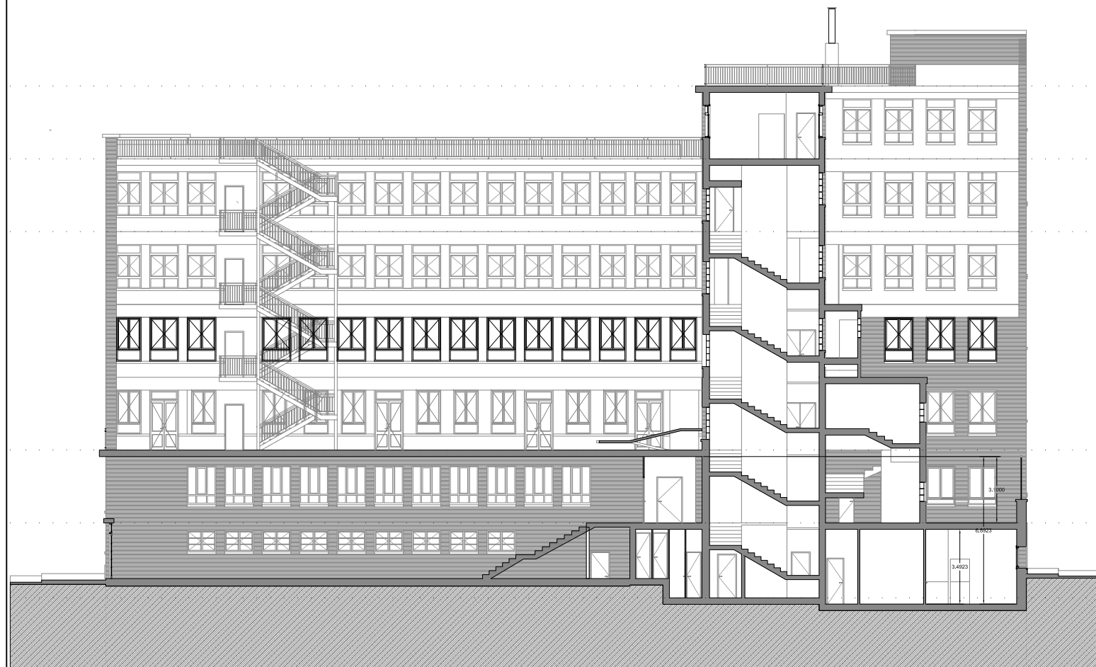
SECCIÓ C-C'
