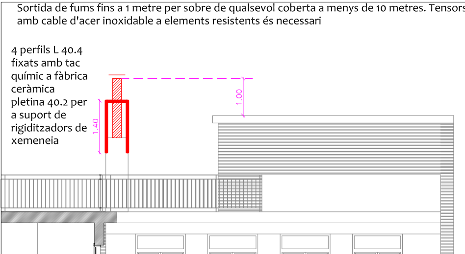
Tram superior de sortida de fums
