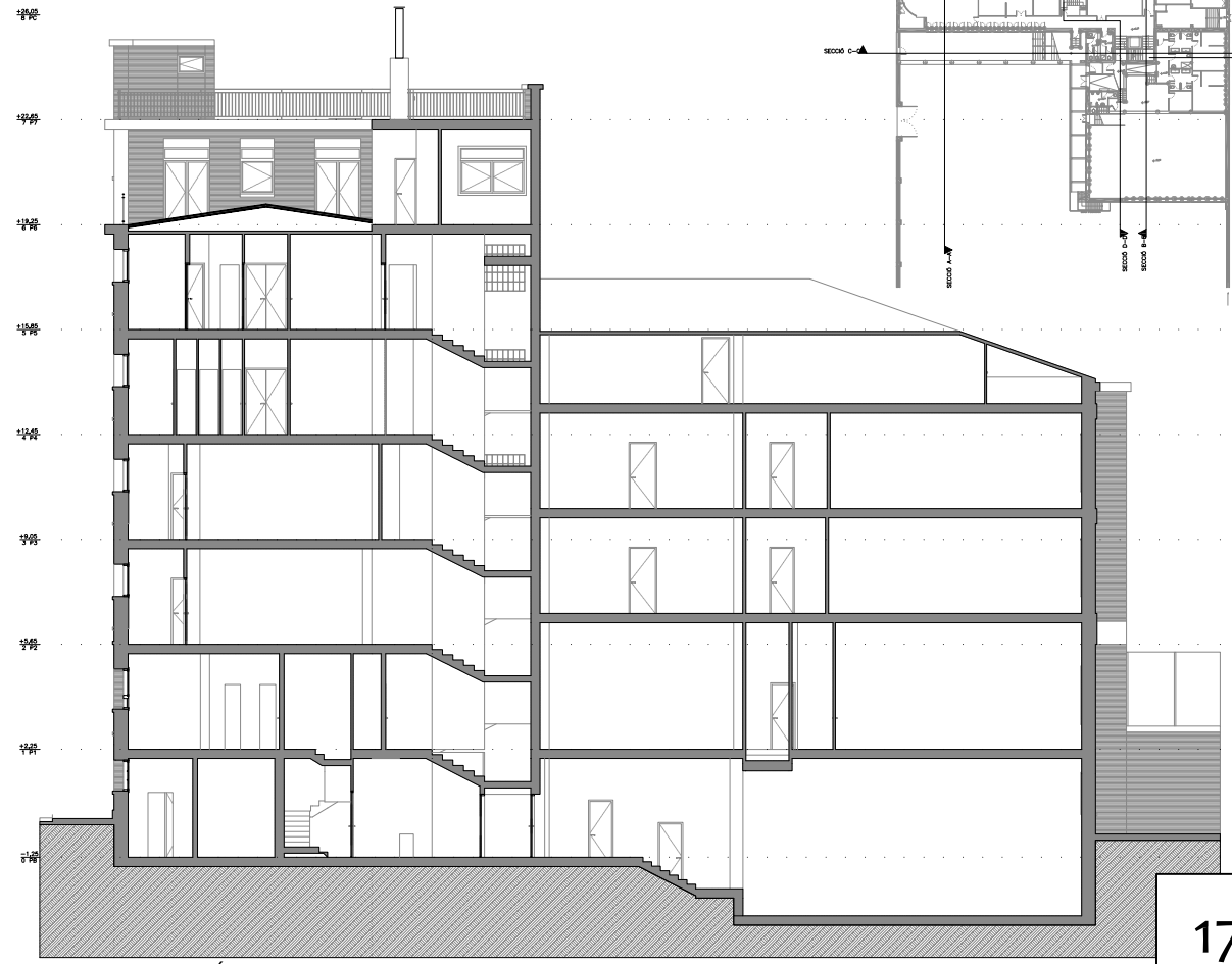
SECCIÓ D-D'
