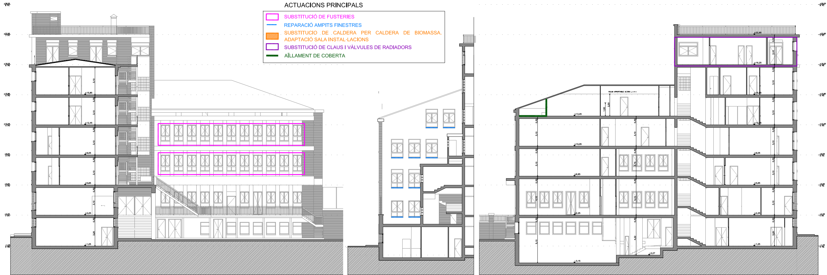
SECCIÓ E-E'
