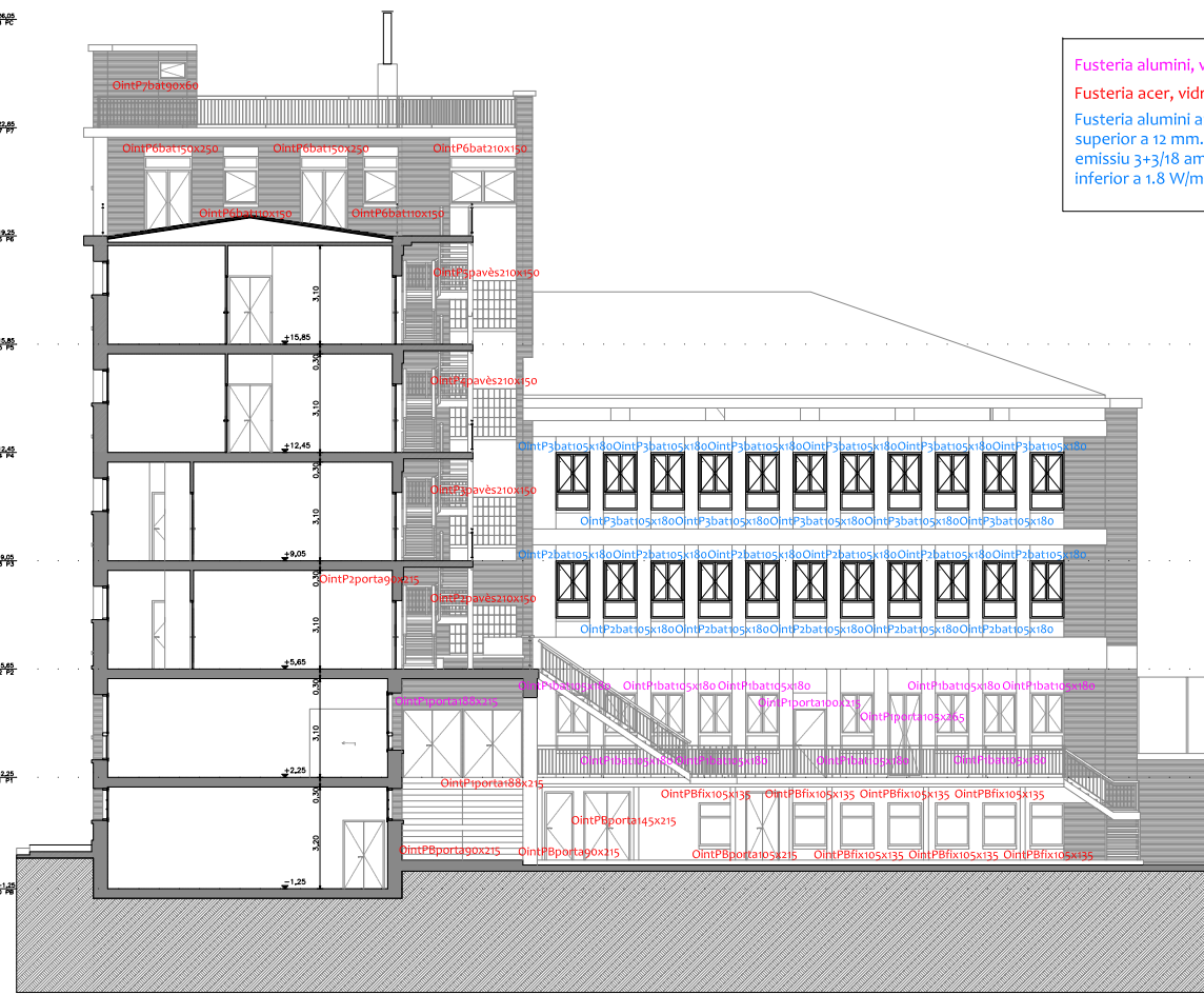
SECCIÓ A-A'
