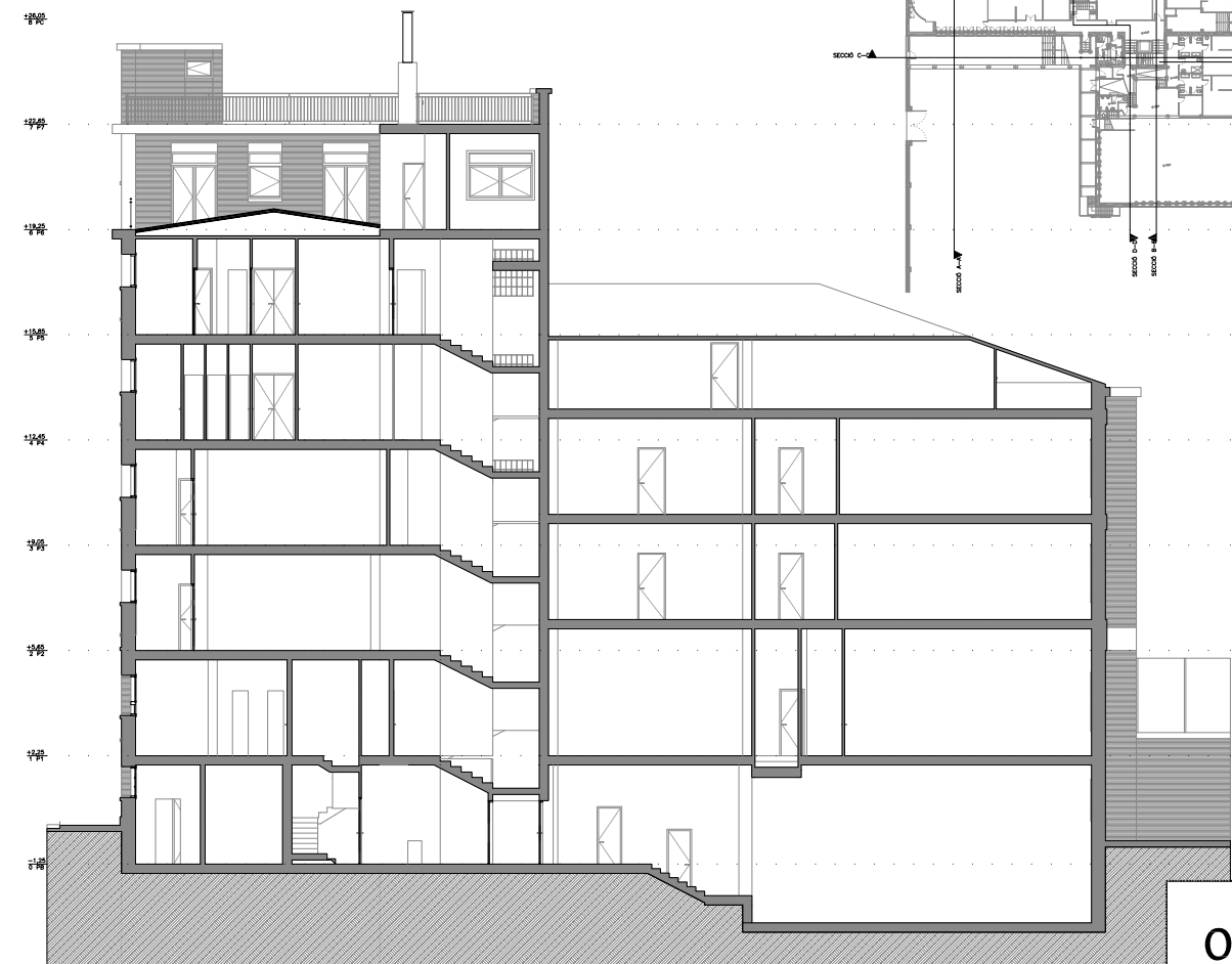
SECCIÓ D-D'
