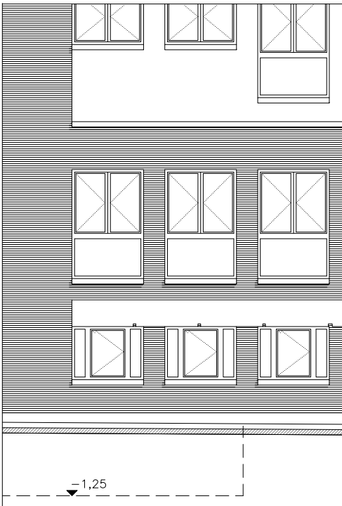
Façana 2. Avinguda Pirineus
