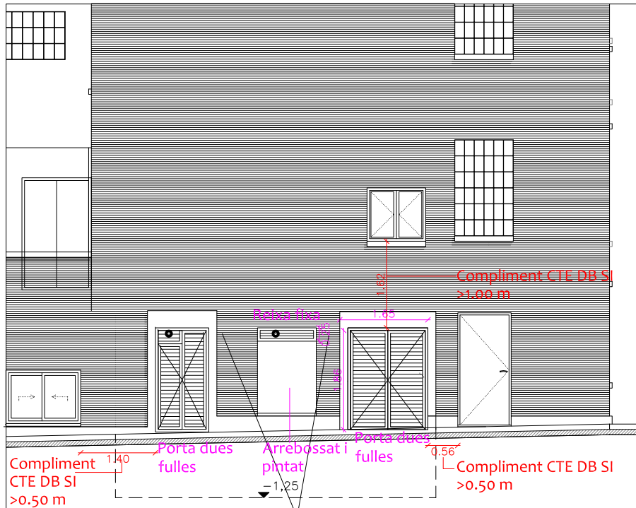
Façana 1. Avinguda Madrid
