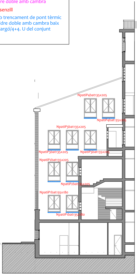
SECCIÓ E-E'
