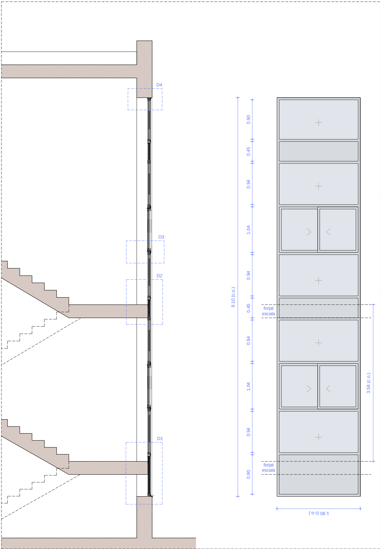
ALÇAT I SECCIÓ ESCALA e 1/50
