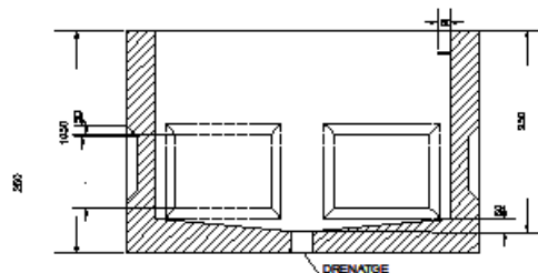
SECCIÓ C-D
