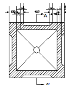
SECCIÓ B-B'
