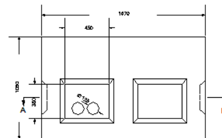
Pericó Tipus C
