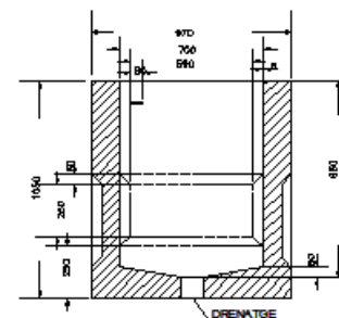
SECCIÓ E-F
