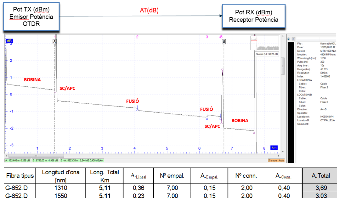
Exemple de mesures òptiques (gràfica reflectometria i taula de potències i atenuacions permeses).
