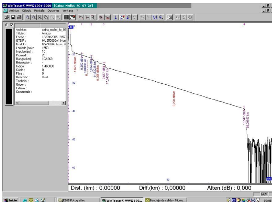
Exemple de gràfica de mesura OTDR.
