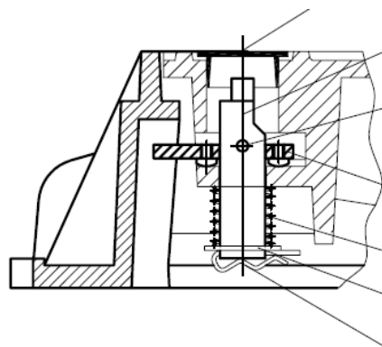
Exemple tanca de seguretat pericó Tipus B/C
