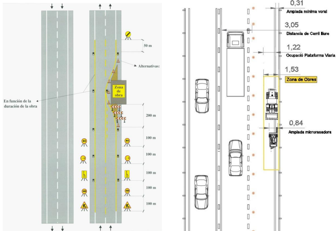
Senyalització per a tall de carril segons 8.3 IC de Carreteres
