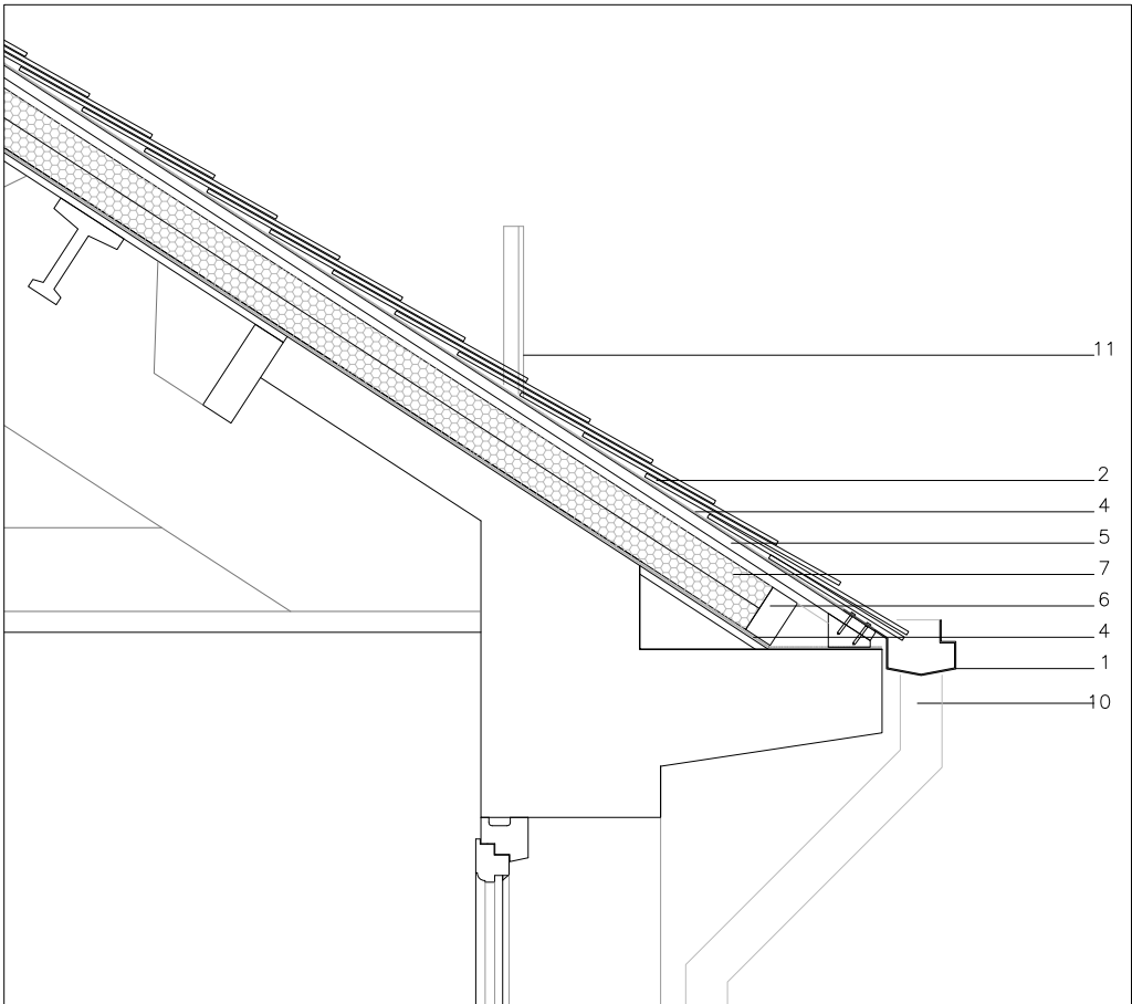
DETALL RÀFEC
