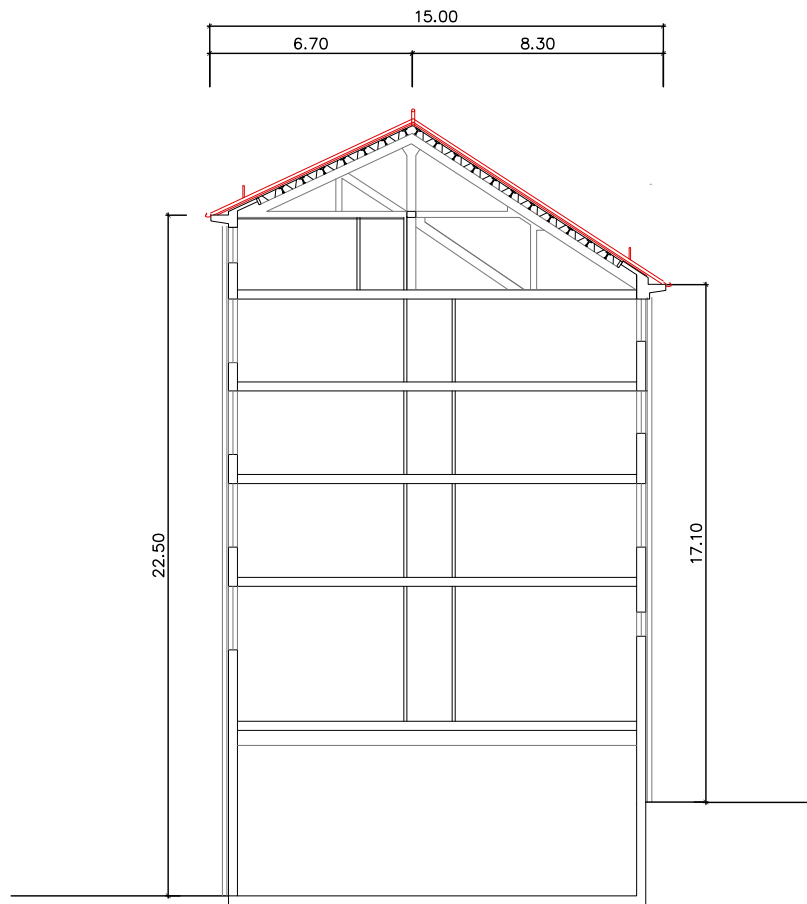
SECCIÓ TRANSVERSAL C-C'
