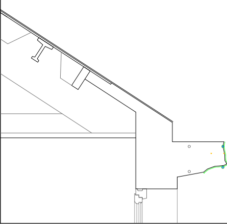
IMPRIMACIÓ AMB REVESTIMENT ANTI-CORROSIÓ I PASSIVADOR SOBRE LES ARMADURES. PONT D'UNIÓ D'ADHERÈNCIA AL FORMIGÓ.
