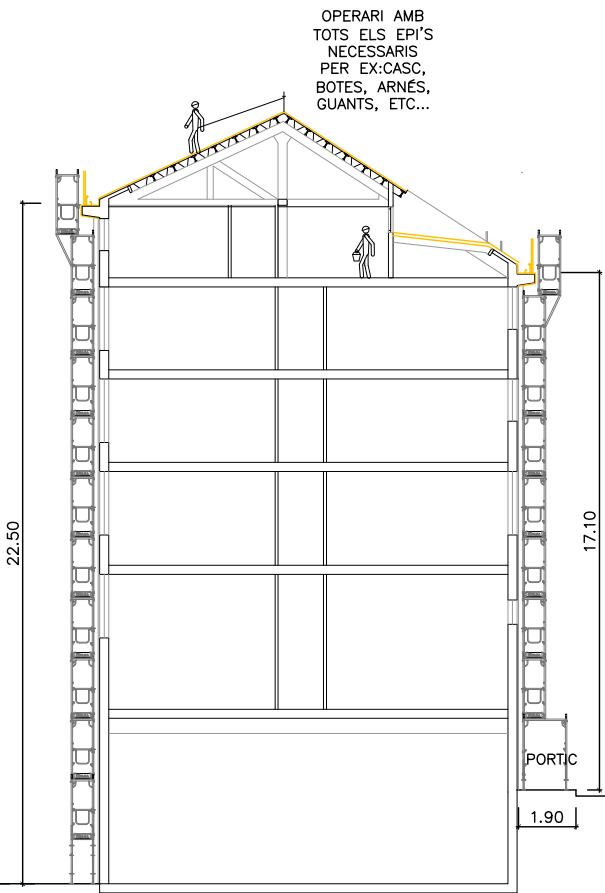
SECCIÓ TRANSVERSAL D-D'
