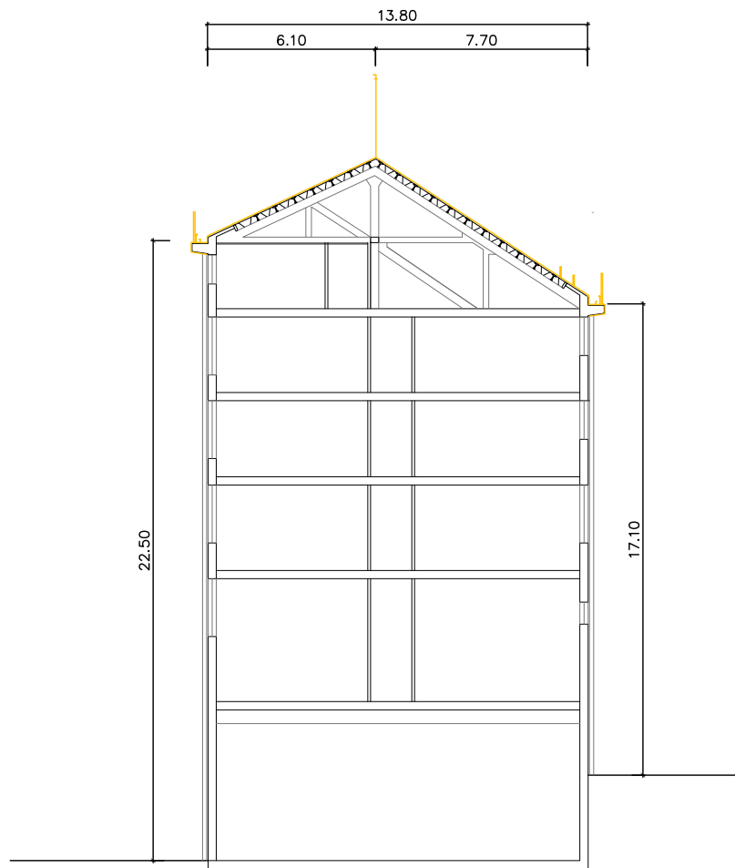
SECCIÓ TRANSVERSAL C-C'
