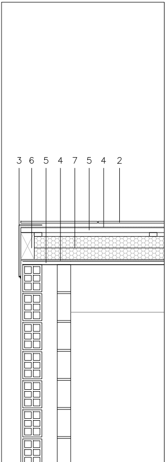
DETALL SUPERIOR FAÇANA LATERAL
