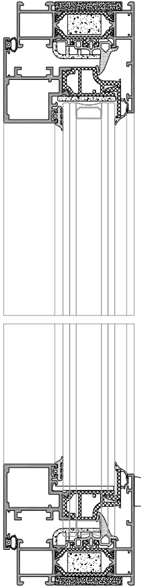
SECCIÓ PERFIL
