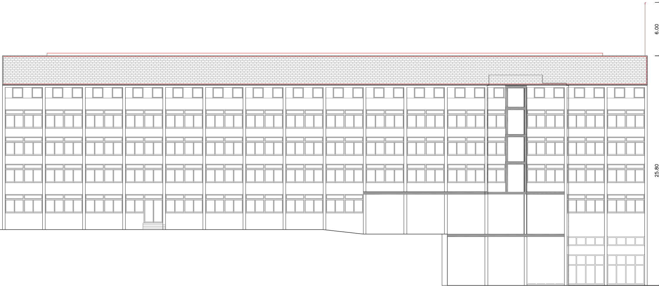
FAÇANA PATI A-A'
