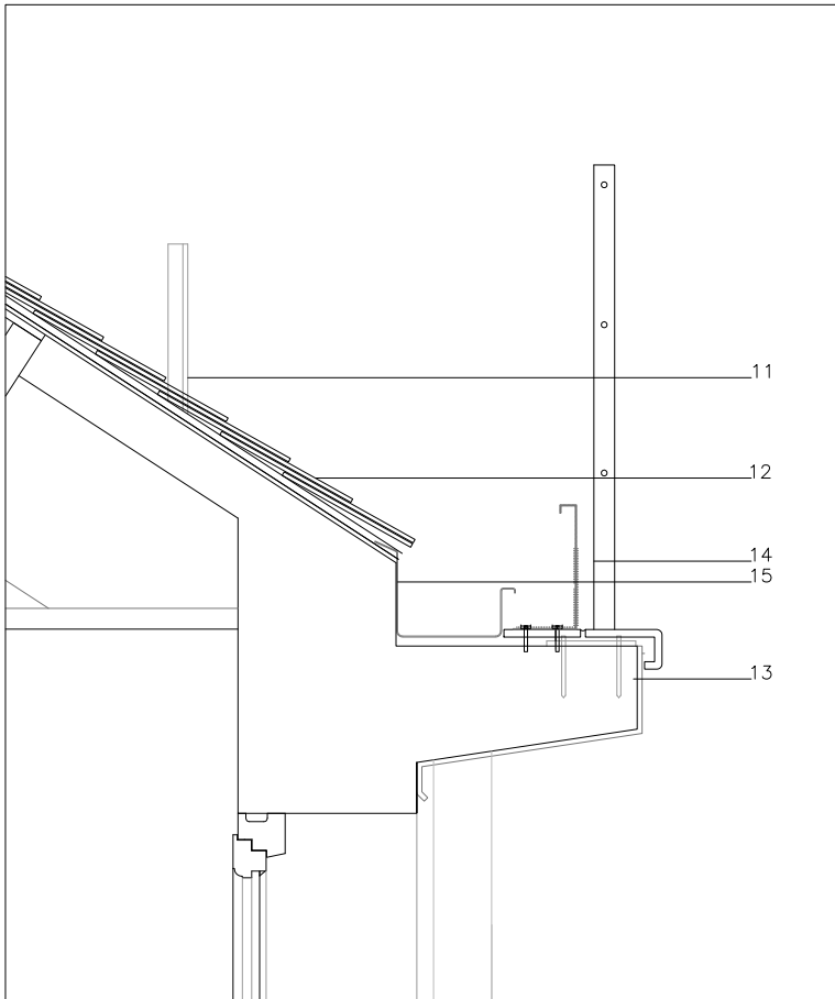
DETALL ESTAT ACTUAL RÀFEC
