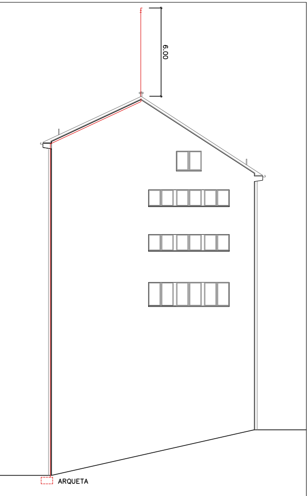
TRAÇAT CABLEJAT INSTAL·LACIÓ PARALLAMPS
