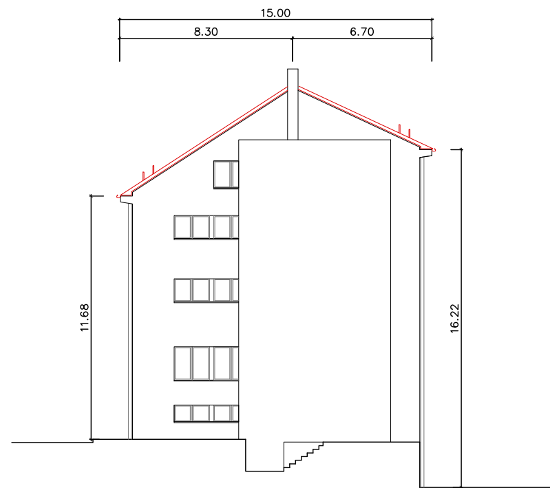
SECCIÓ TRANSVERSAL D-D'
