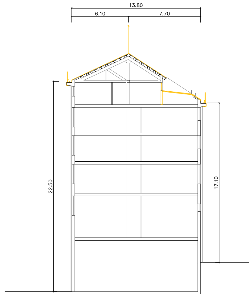
SECCIÓ TRANSVERSAL D-D'
