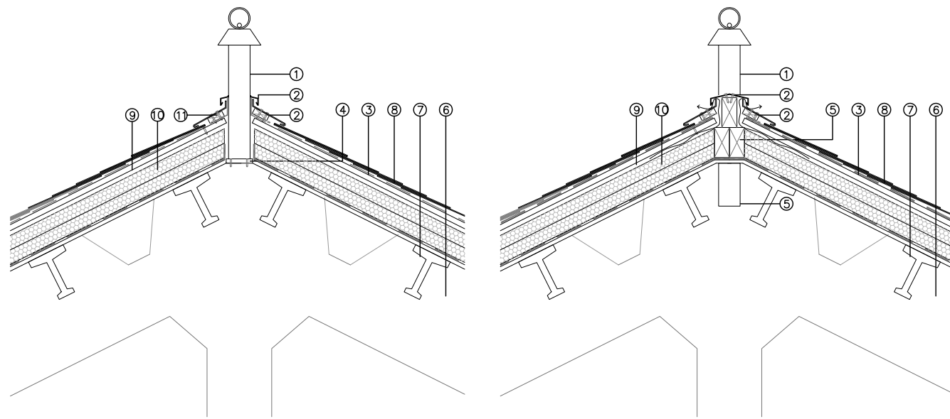
DETALL LINIA DE VIDA I CARENER
