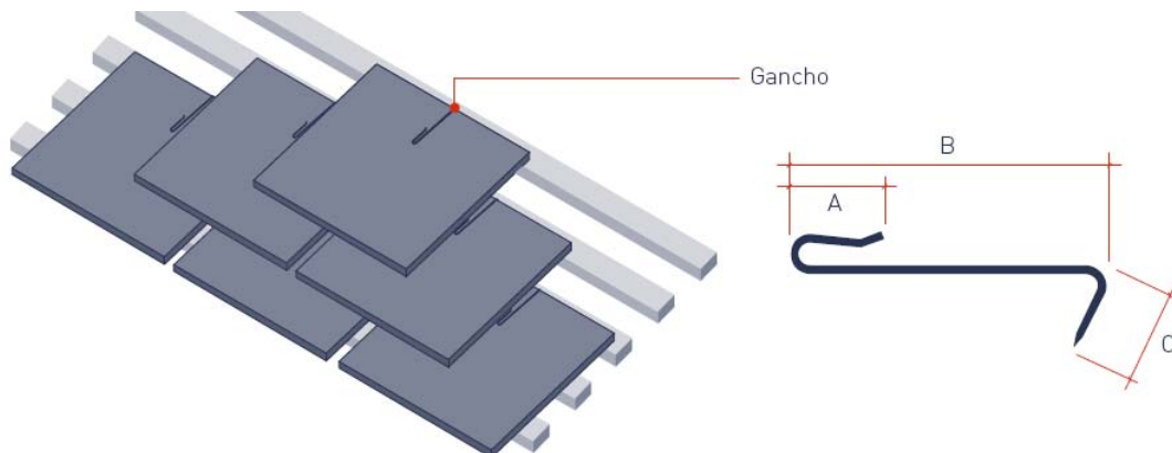
Esquema muntatge pissarra amb ganxos
