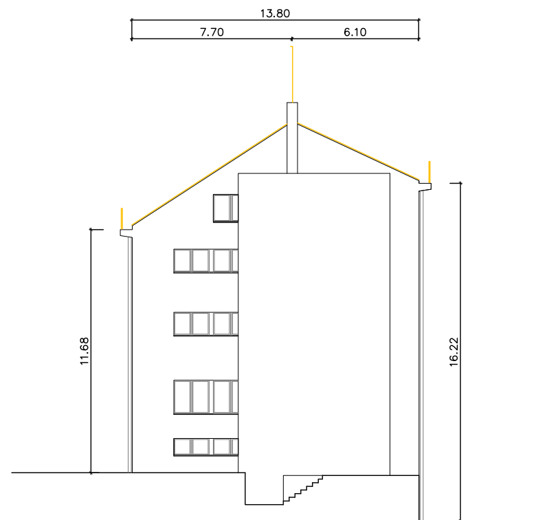
SECCIÓ TRANSVERSAL D-D'
