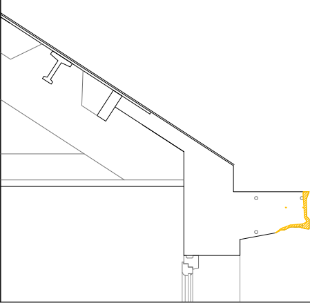
REPICAT I SANEJAT DEL FORMIGÓ DEFECTUÓS
