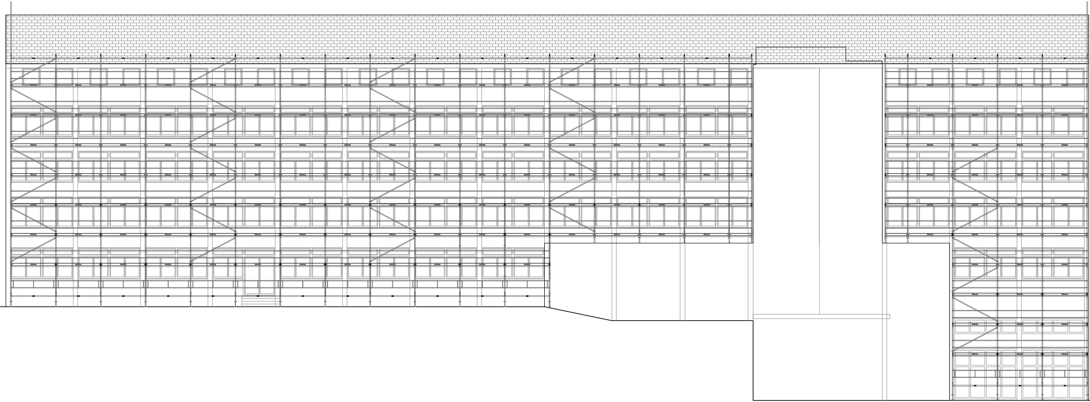
FAÇANA PATI A-A'
