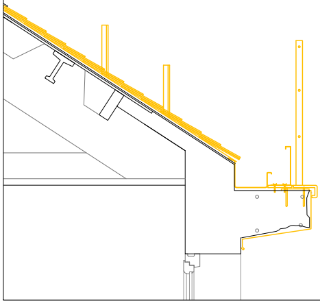
EXTRACCIÓ DE PEÇA DE PISSARRA, PEÇA DE REMAT, CANAL, BARANA
