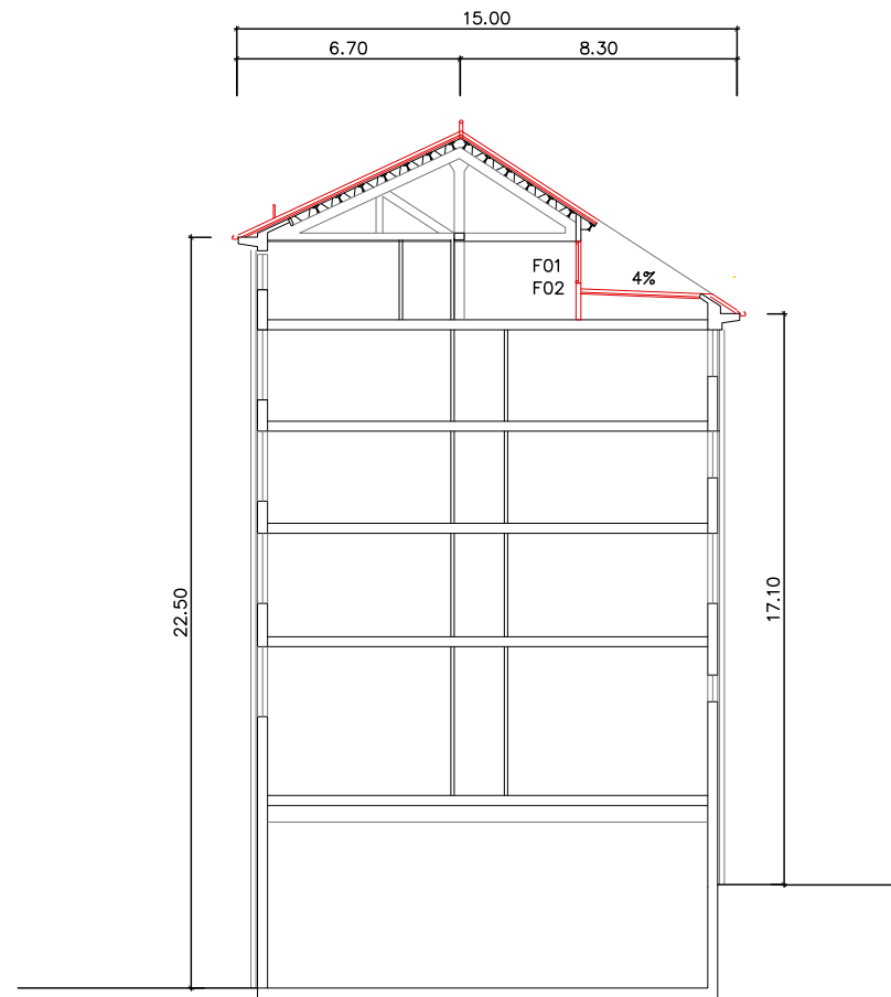
SECCIÓ TRANSVERSAL D-D'
