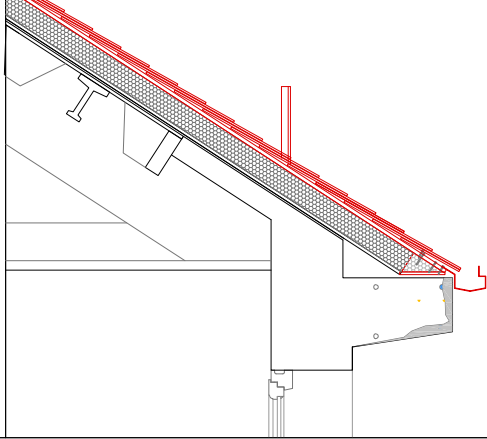
RECONSTRUCCIÓ AMB MORTER HIDRÒFUG D'ALTA RESISTÈNCIA I BAIXA RETRACCIÓ. FORMACIÓ DE COBERTA
