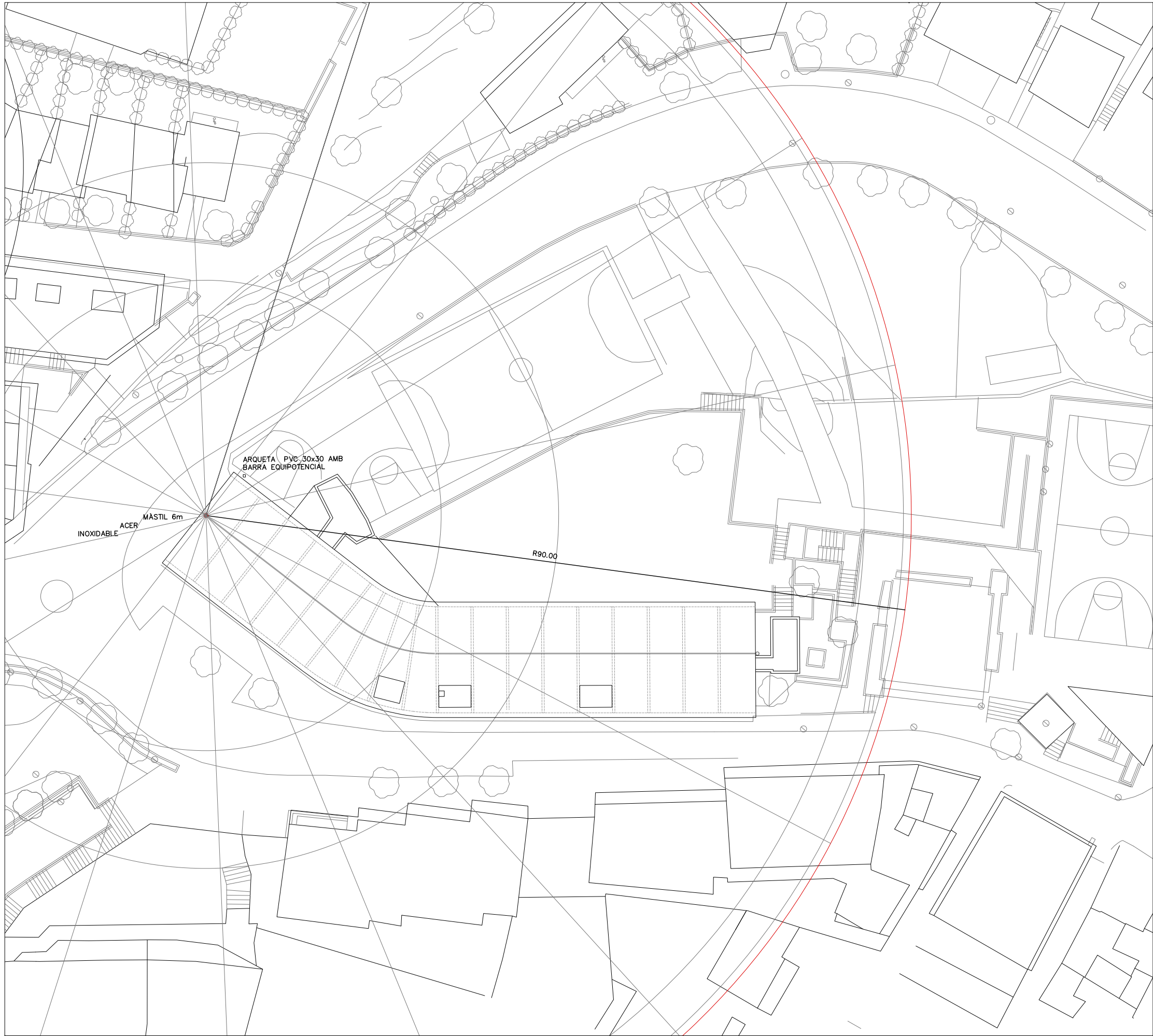
TRAÇAT CABLEJAT INSTAL·LACIÓ PARALLAMPS
