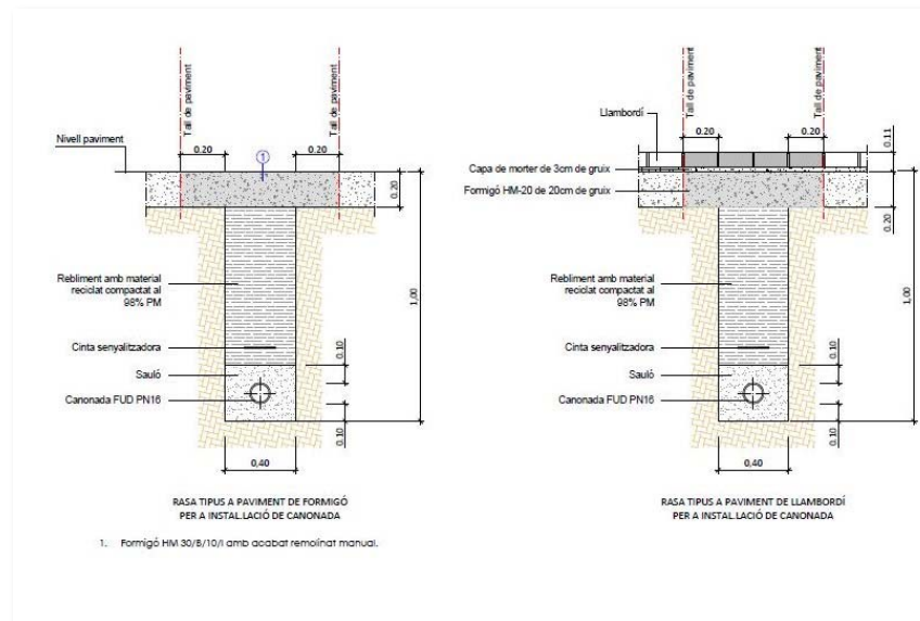
Rases tipus calçada
