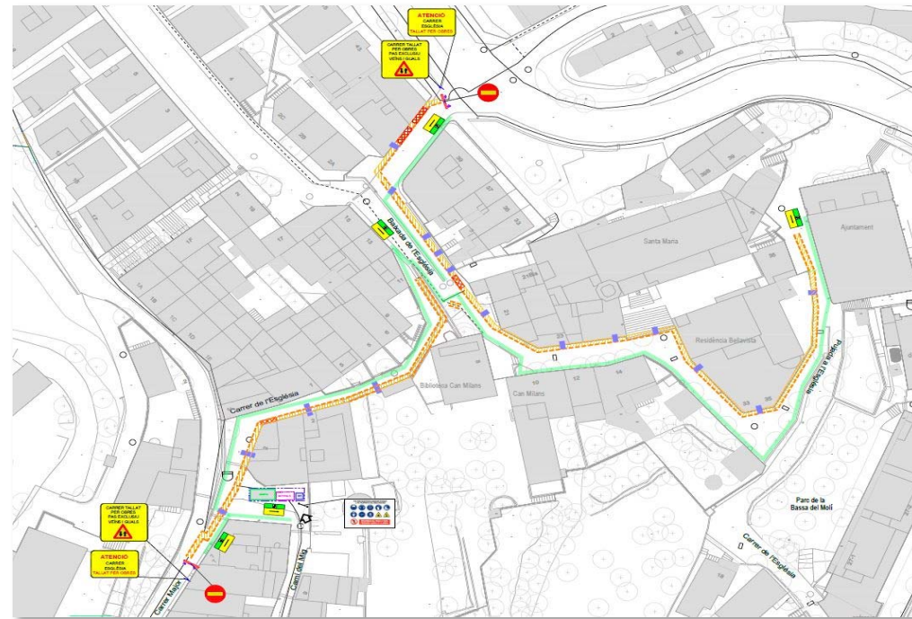
Implantació de les obres proposada
