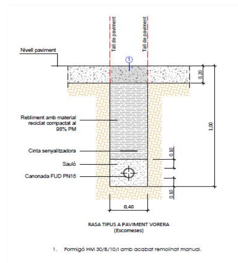
Rases tipus per escomeses
