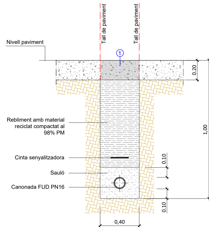
RASA TIPUS A PAVIMENT VORERA (Escomeses)
