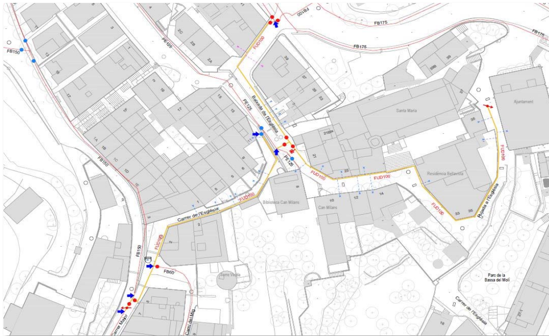
Xarxa d'aigua potable existent
