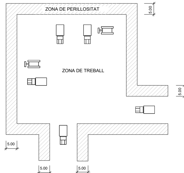
DETALL Delimitació zones de treball ESCALA 5/E
