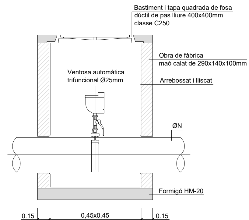
DETALL ARQUETA VÀLVULA VENTOSA
