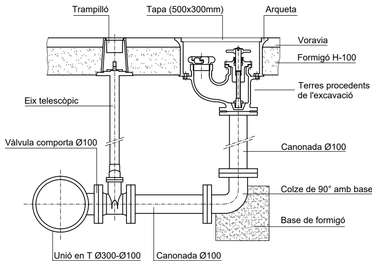
HIDRANT SOTERRAT
