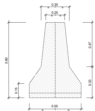
SECCIÓ A-A'
