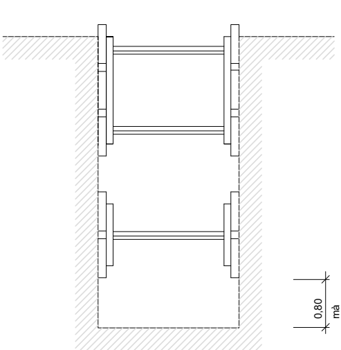
Rases amb apuntalament sense sobrecàrrega
