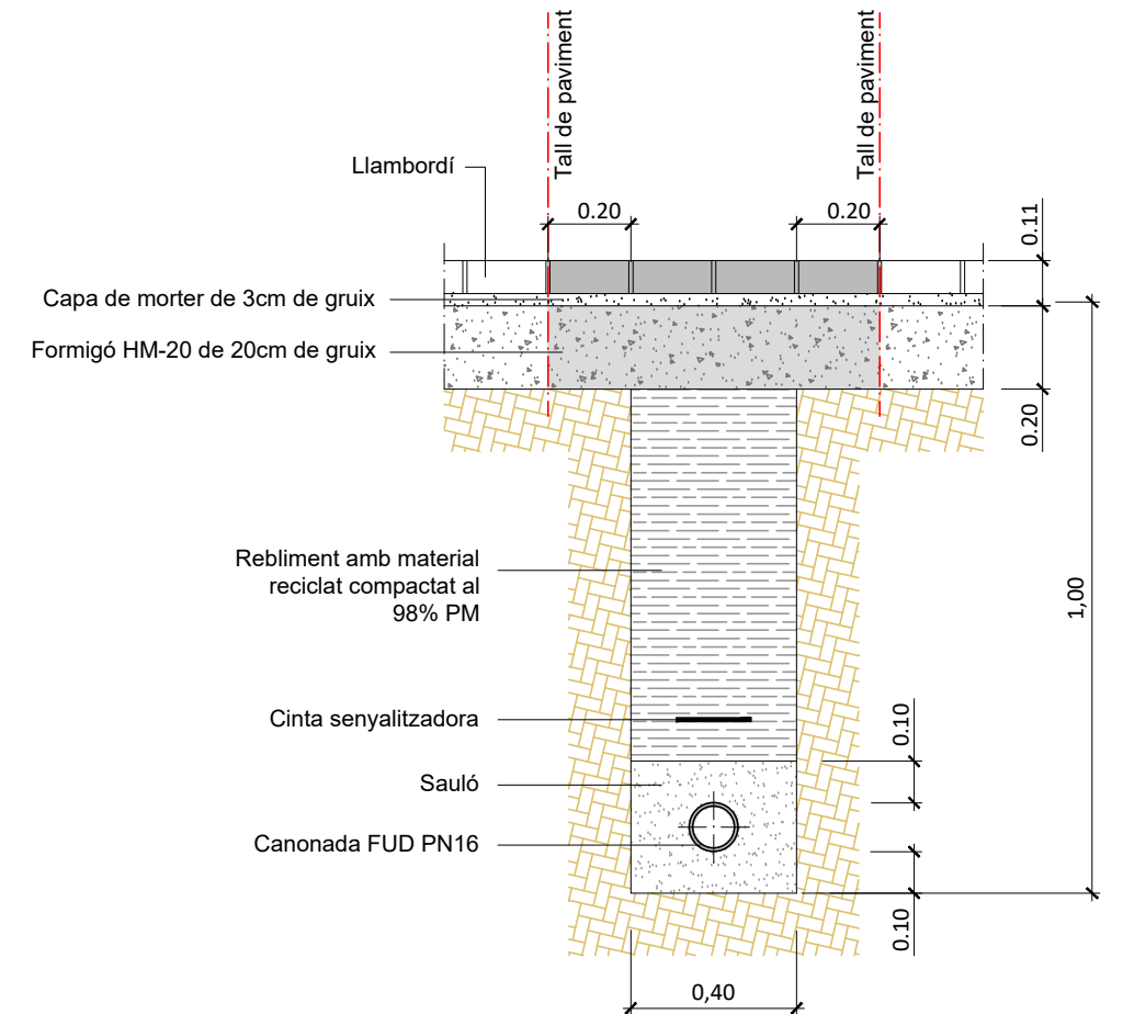
RASA TIPUS A PAVIMENT DE LLAMBORDÍ PER A INSTAL·LACIÓ DE CANONADA
