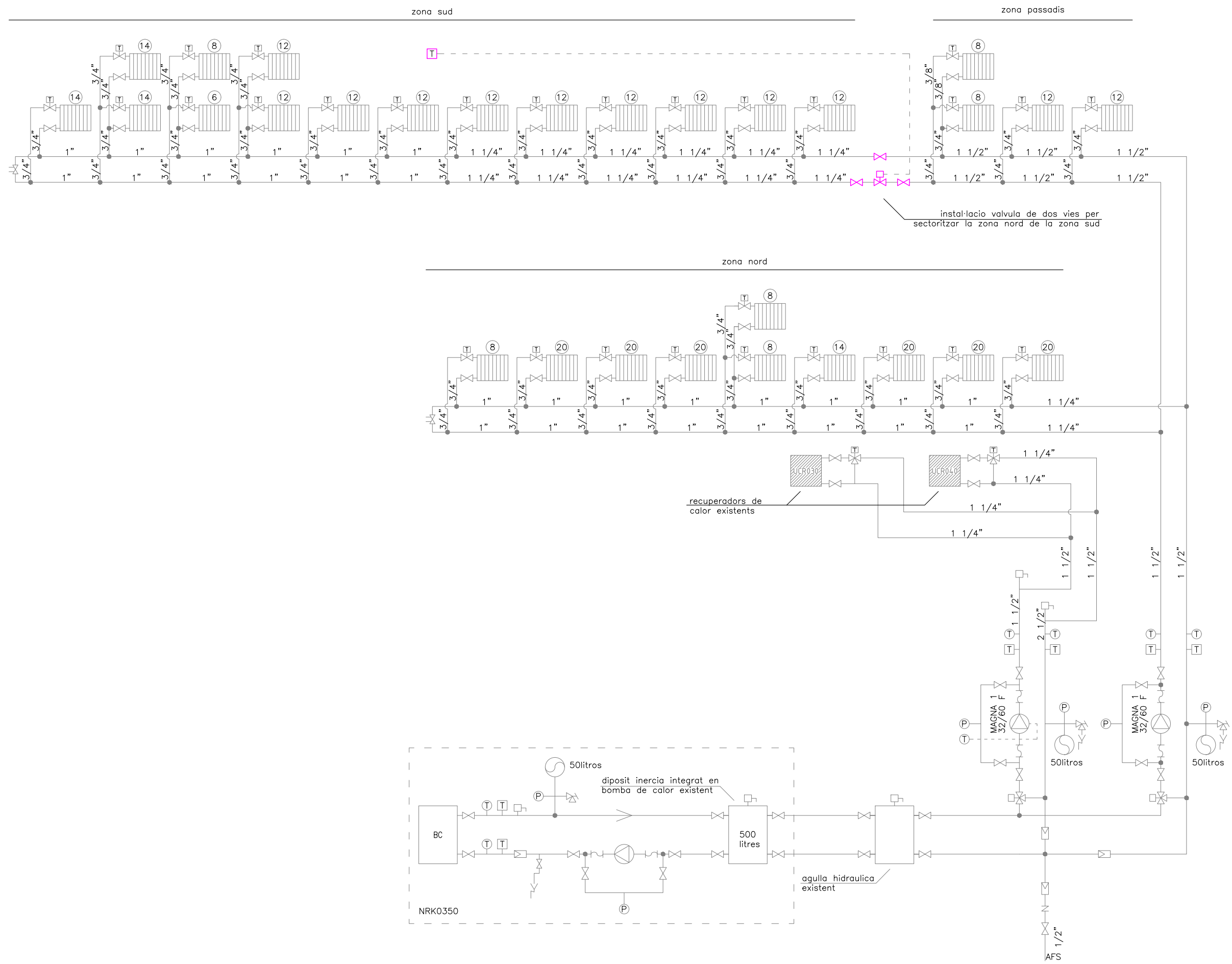
Climatitzacio. Circuit hidraulic. Tuberies.
