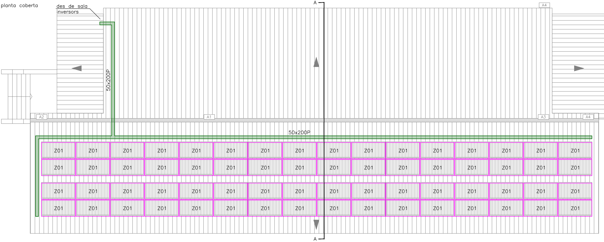
planta coberta
