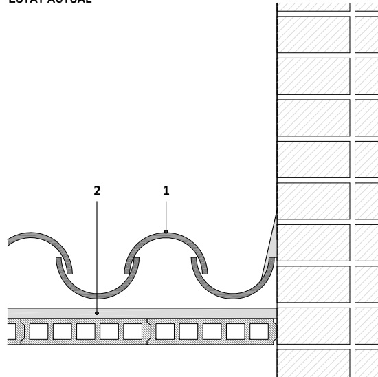
ESTAT ACTUAL
