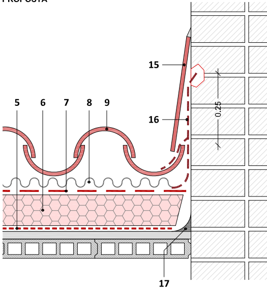
PROPOSTA
