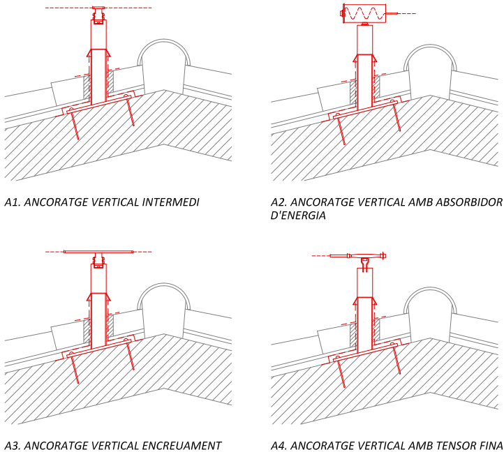
DETALL ANCORATGES DE LINIA DE VIDA e.1:20
