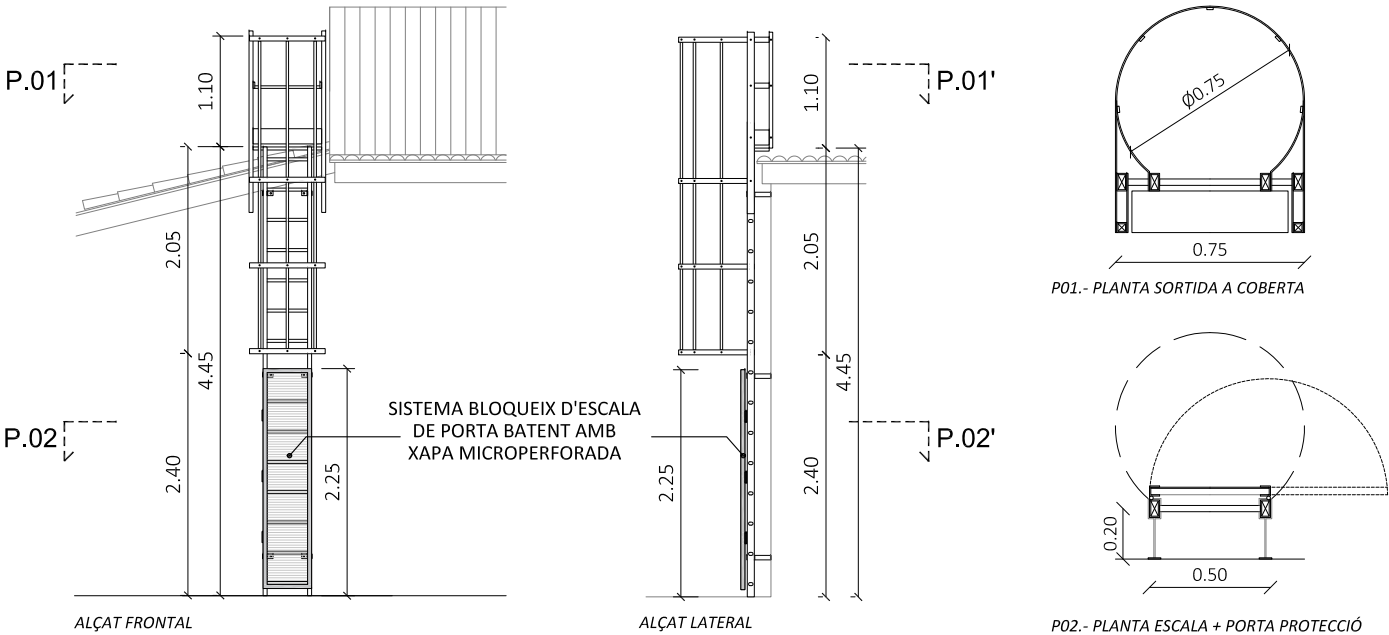
DETALL ESCALA DE GAT AMB SISTEMA DE BLOQUEIX e.1:75
