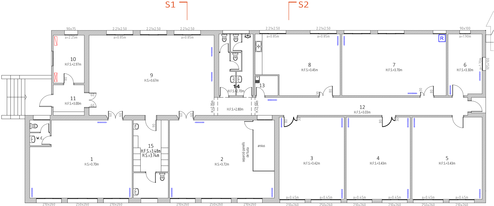
PLANTA BAIXA
