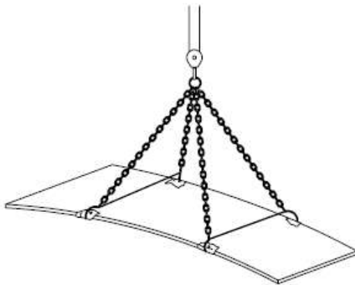
CARREGA LLARGA AMB DUES ESLINGAS
