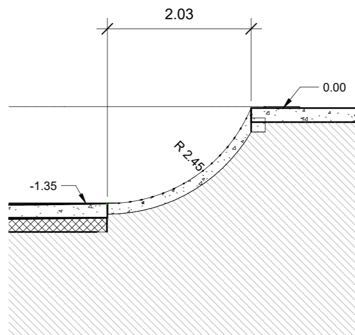
4 seccion 6 1 : 50
