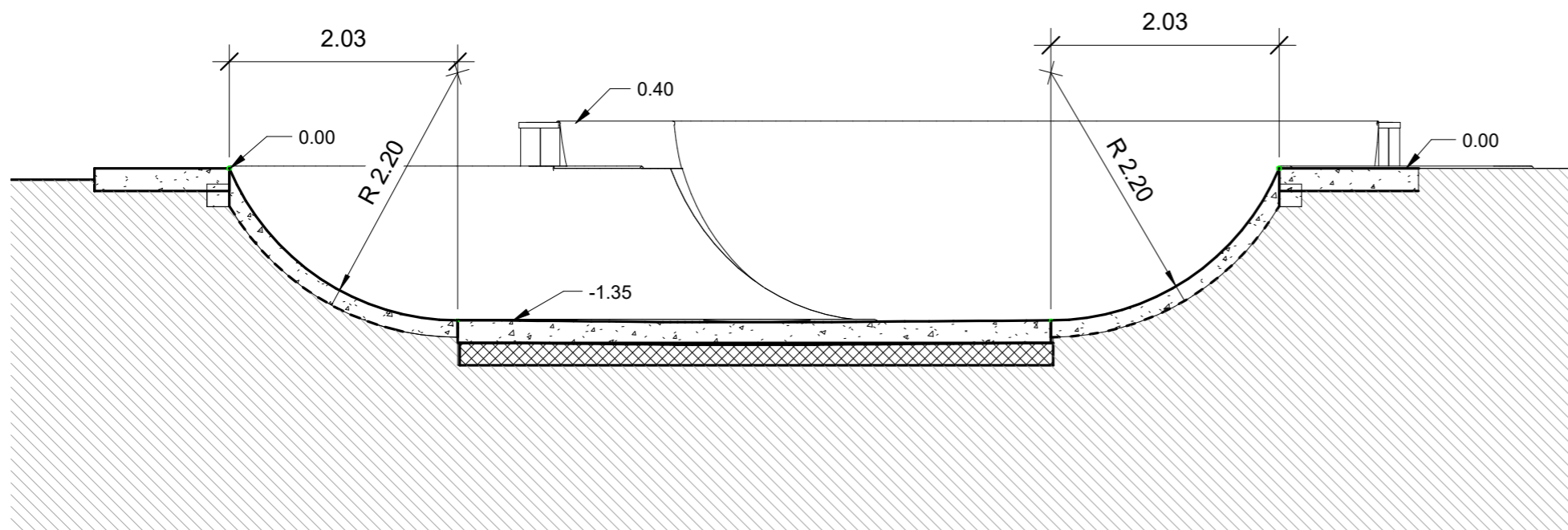
2 seccion 4 1 : 50
