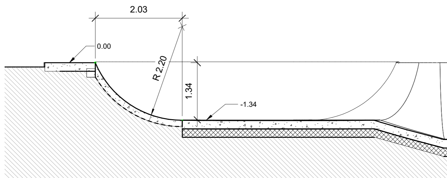
2 seccion 1 1 : 50
