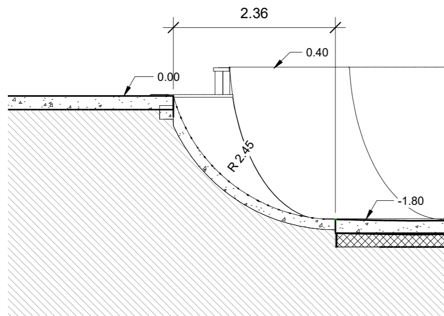
3 seccion 5 1 : 50
