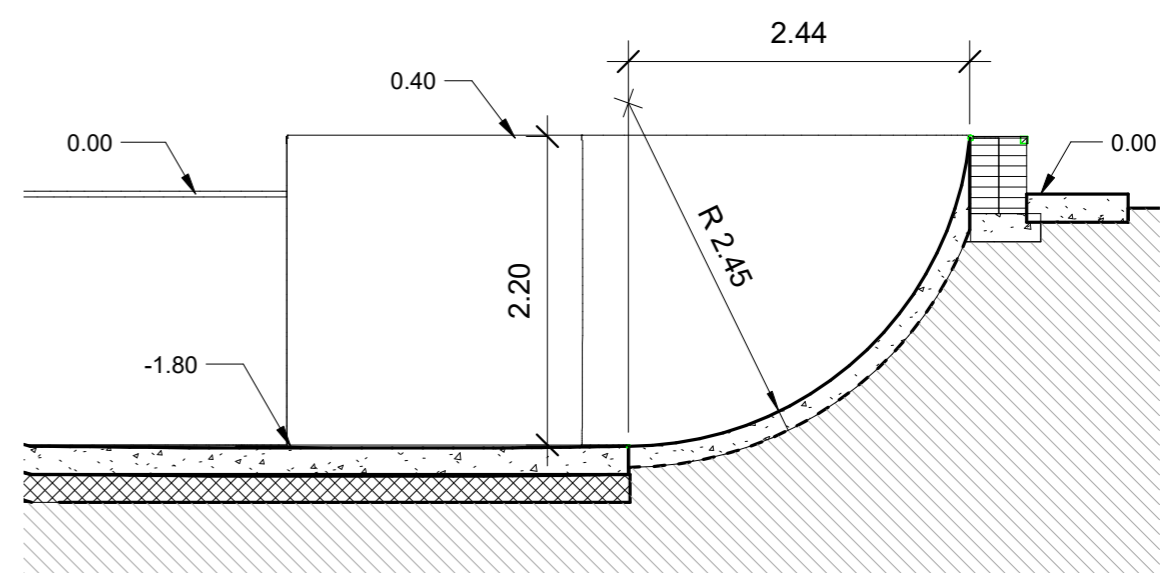
3 seccion 2 1 : 50
