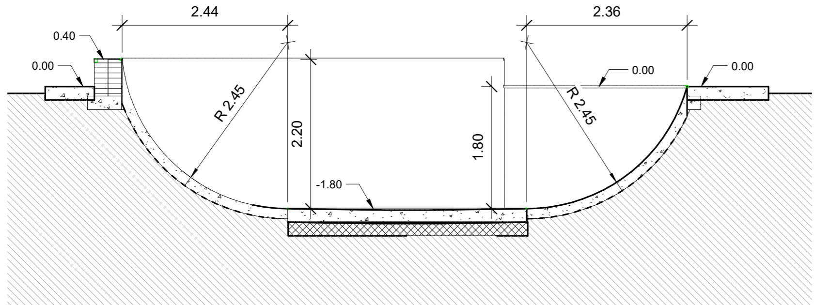
4 seccion 3 1 : 50
