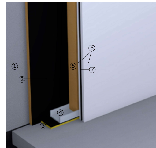
DETALL Y - Revestiment parets mitgeres (Trasdossat A)
