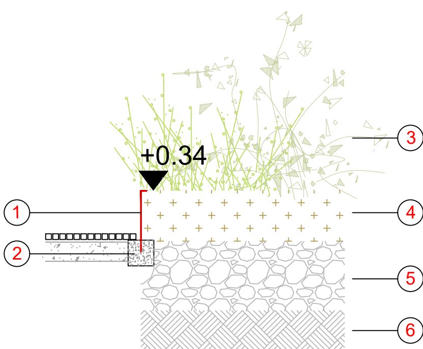
DETALL JARDINERA D'ACER CORTEN
