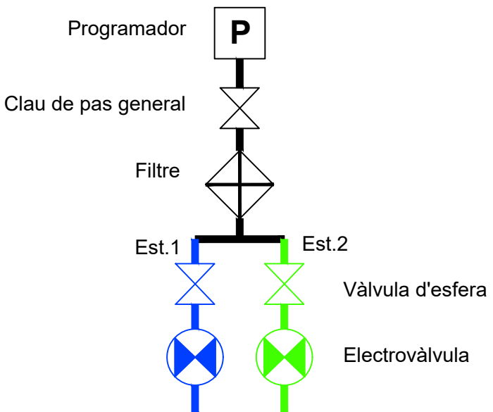
ESQUEMA INSTAL·LACIÓ DE REG
