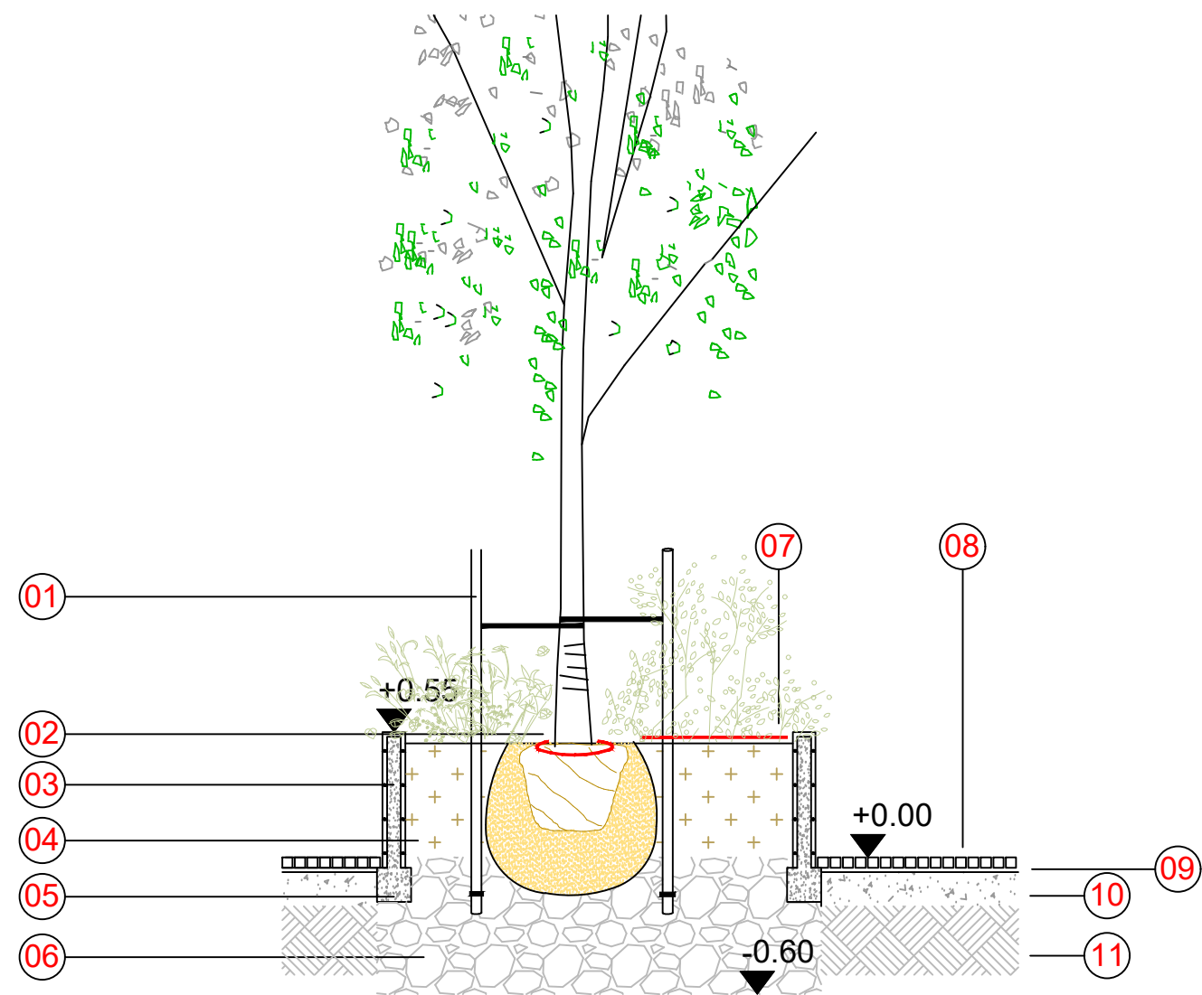
DETALL JARDINERA DE FORMIGÓ
