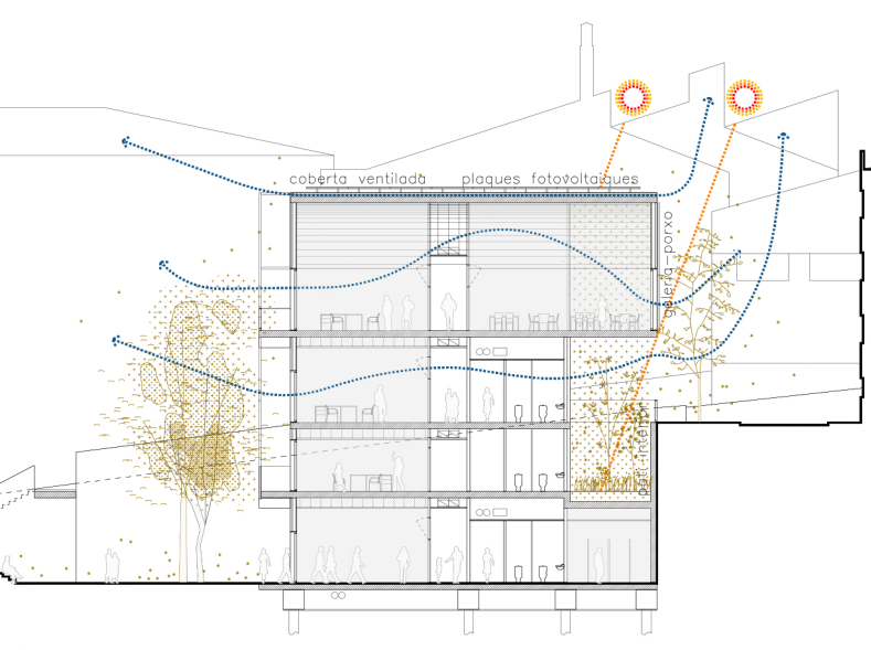
> Secció transversal | e:1/400
