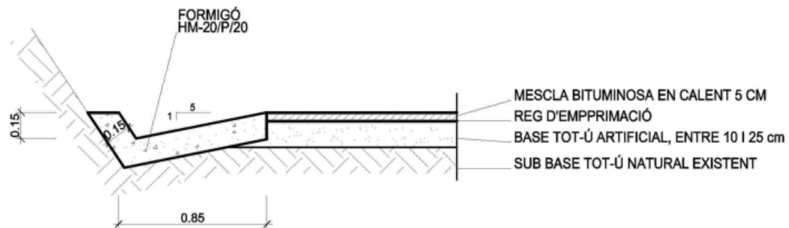
DETALLS CUNETAS ESCALA 1/50
