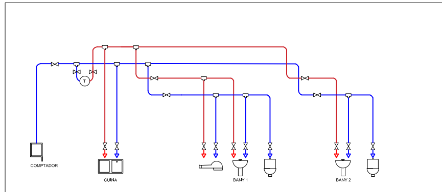
ESQUEMA HIDRÀULIC_PIS_TIPUS_B
