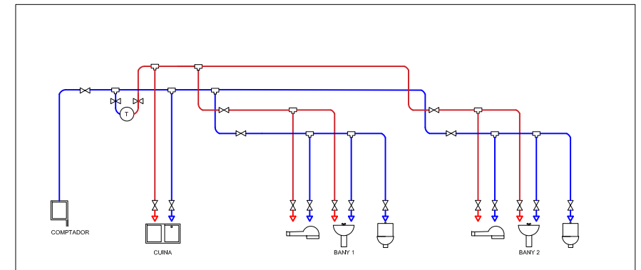
ESQUEMA HIDRÀULIC_PIS_TIPUS_C
