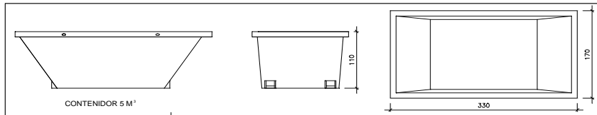
CONTENIDOR 5 M 3
