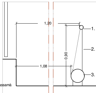
SECCIÓ A
