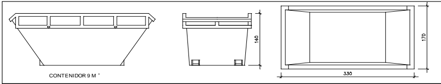
CONTENIDOR 9 M 3
