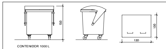
CONTENIDOR 1000 L
