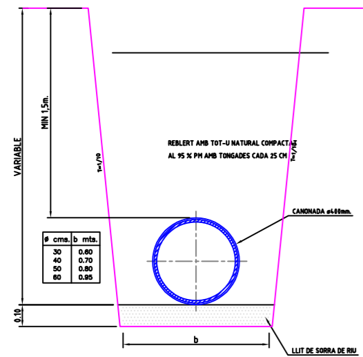
RASA TIPUS
