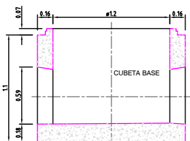
POU DE REGISTRE
