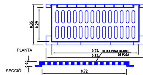
REIXA I MARC D'EMBORNAL
