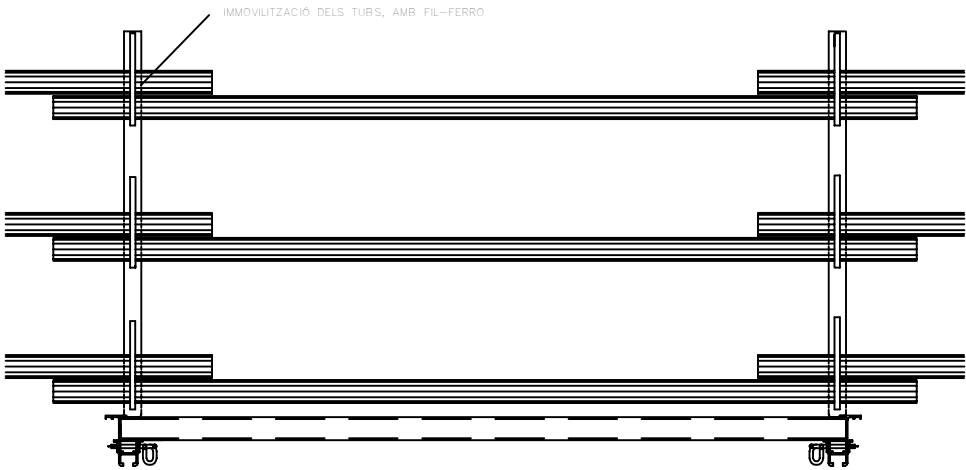
ALÇAT ESCALA 1/10
