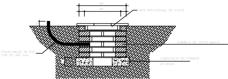
ALÇAT
