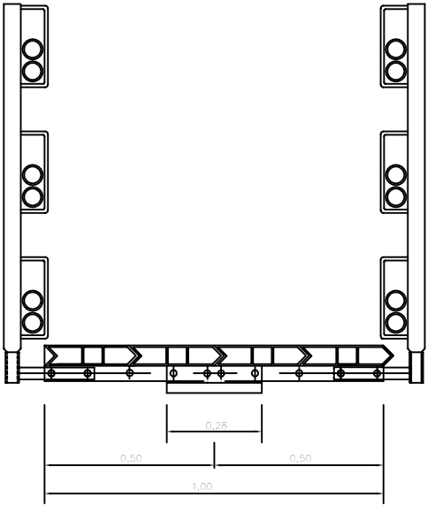
SECCIÓ ESCALA 1/10
