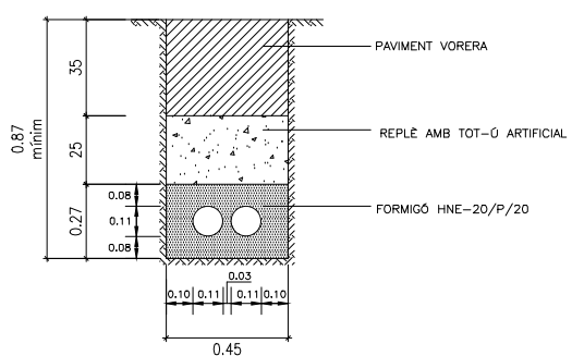
RASA TIPUS SOTA VORERA TELECOMUNICACIONS 2 COND. DE PVC Ø110 gruix=1,2 mm
