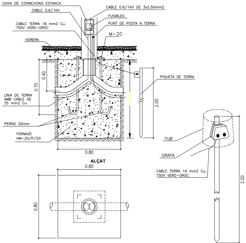
PLANTA FONAMENTACIÓ PUNTS DE LLUM
