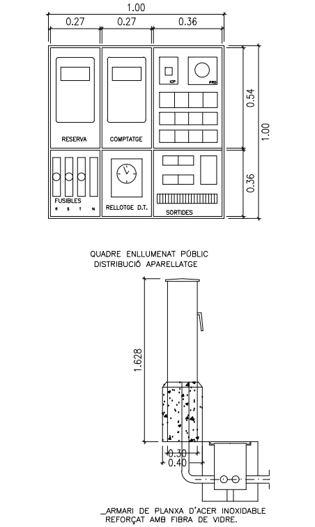
QUADRE ENLLUMENAT PÚBLIC
