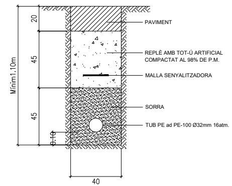
RASA EN VORERA AIGUA TUB P.E. a.d. Ø32mm PN16
