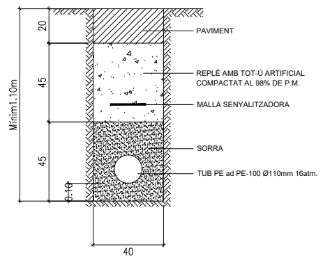
RASA EN VORERA AIGUA TUB P.E. a.d. Ø110mm PN16
