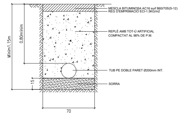
RASA EN CALÇADA DRENATGE
