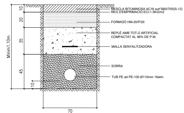
RASA EN CALÇADA AIGUA TUB P.E. a.d. Ø110mm PN16
