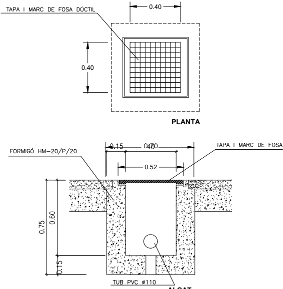
ARQUETA DE REGISTRE
