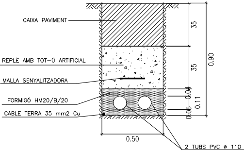
RASA ENLLUMENAT SOTA CALÇADA
