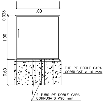
REPEU D'OBRA DE FÀBRICA AMB FORMIGÓ HM-20/P/20 EXTERIOR REMOLINAT.
