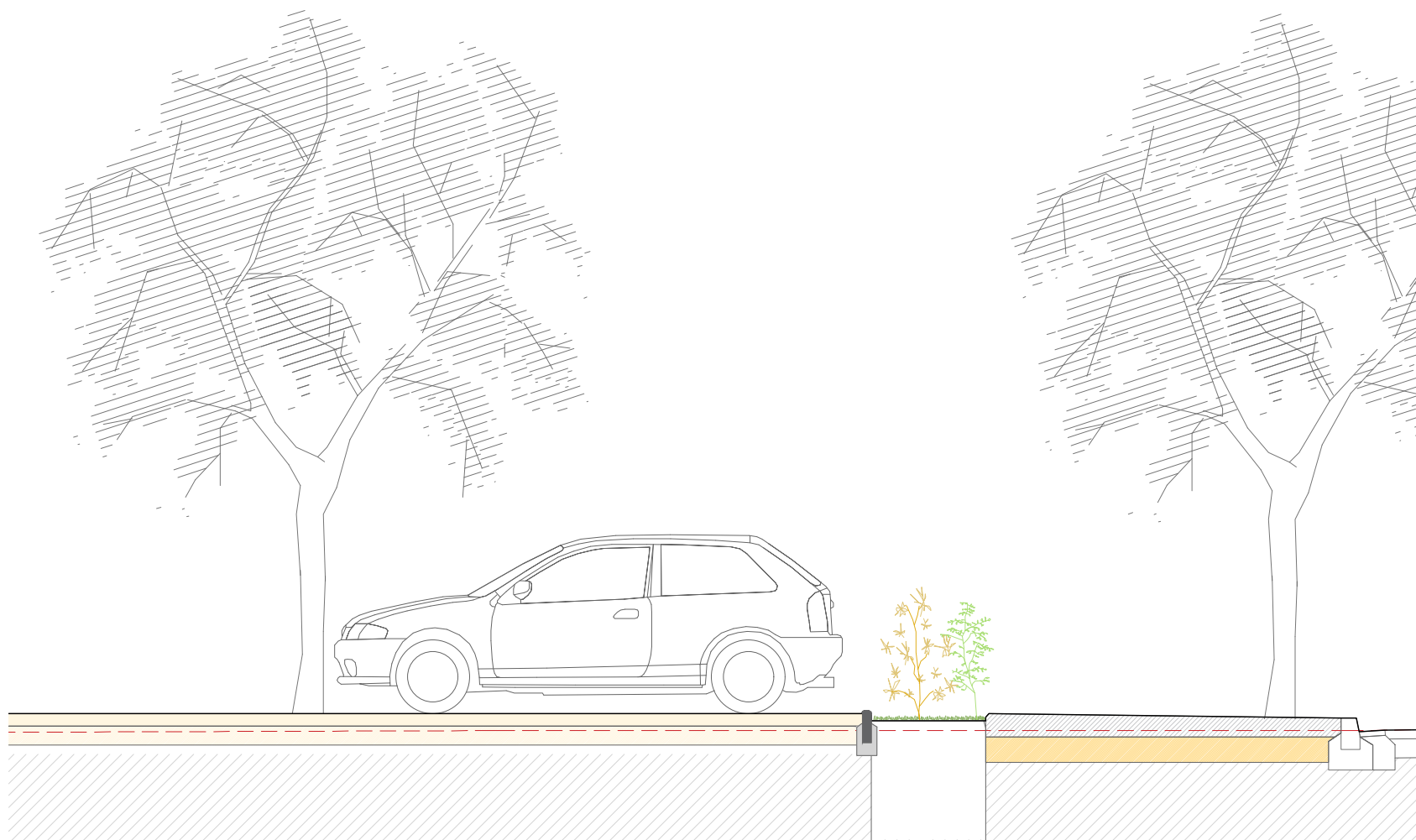
Detall aparcament-vorera
