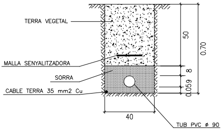
RASA ENLLUMENAT SOTA SAULÓ/TERRES
