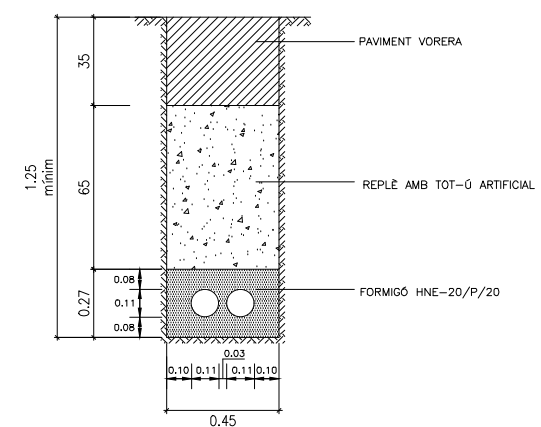
RASA TIPUS SOTA CALÇADA TELECOMUNICACIONS 2 COND. DE PVC Ø110 gruix=1,2 mm
