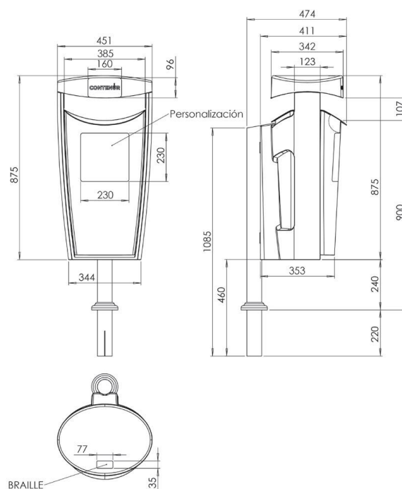
Imatge 2. Esquema constructiu orientatiu amb el sistema de fixació mitjançant poste encastat.
