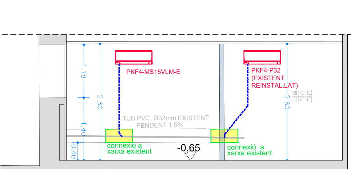
SECCIÓ TRANSVERSAL A-A'
