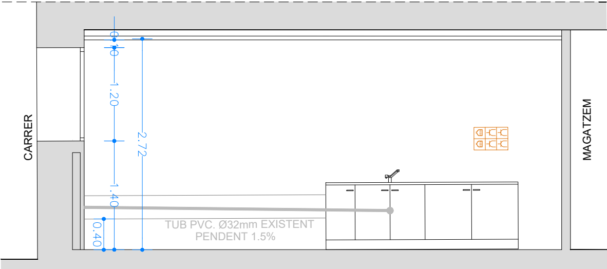
SECCIÓ TRANSVERSAL A-A'
