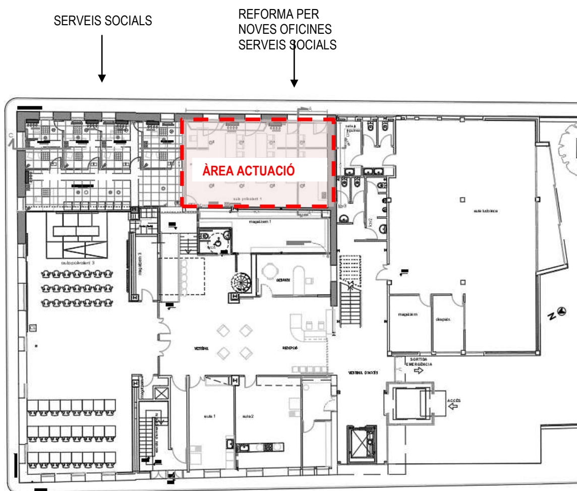
Planta baixa – àrea d'actuació
