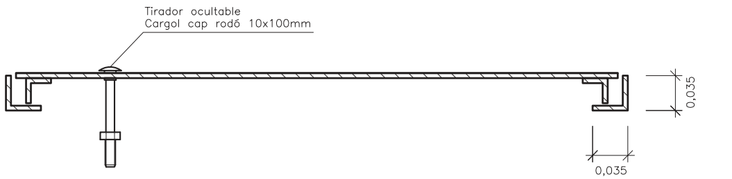
SECCIÓ A–A'
