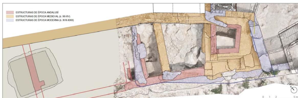
Fig. 3. Cronología provisional atribuida a las estructuras arqueológicas localizadas en el ámbito del bastión.
