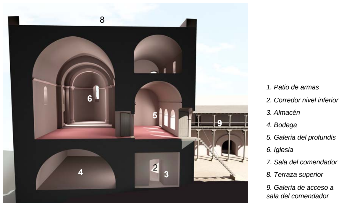
Fig. 5. Sección transversal del cuerpo septentrional del recinto soberano donde se sitúa la sala del comendador.
