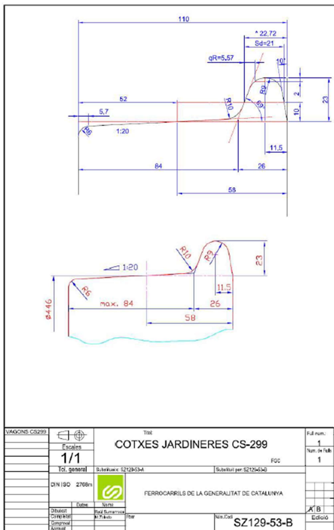
Fig. 27. Cotxes Jardineres Plataforma SCHÖMA CS-299 (CTC1, CTC2, CTC3 i CTC4) (plànol: SZ129-53-B_Cotxes jardineres CS-299.dwg)
