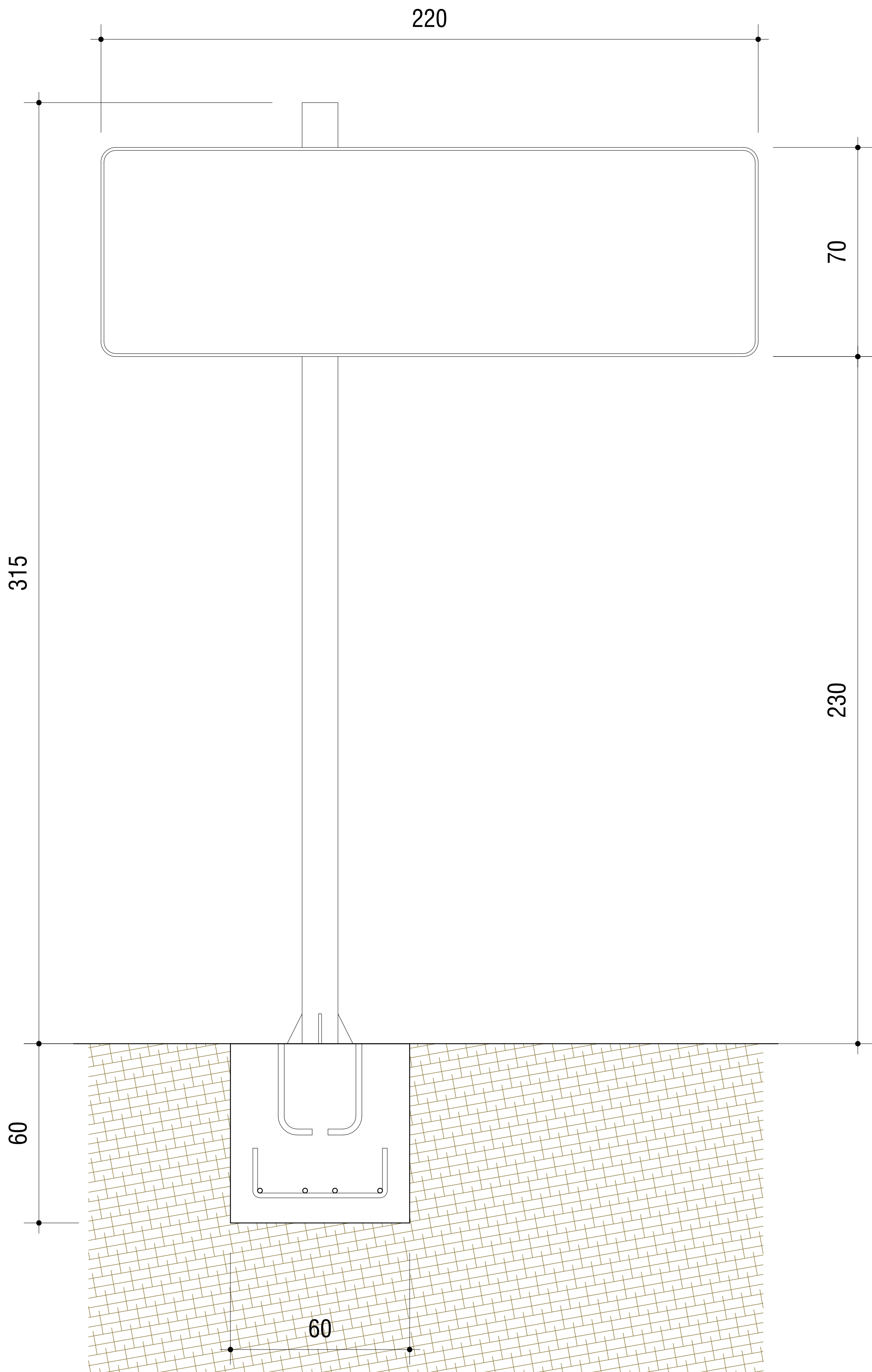
ALÇAT FRONTAL
