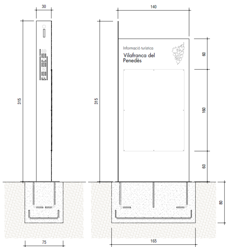
Dibuix alçat lateral i frontal
