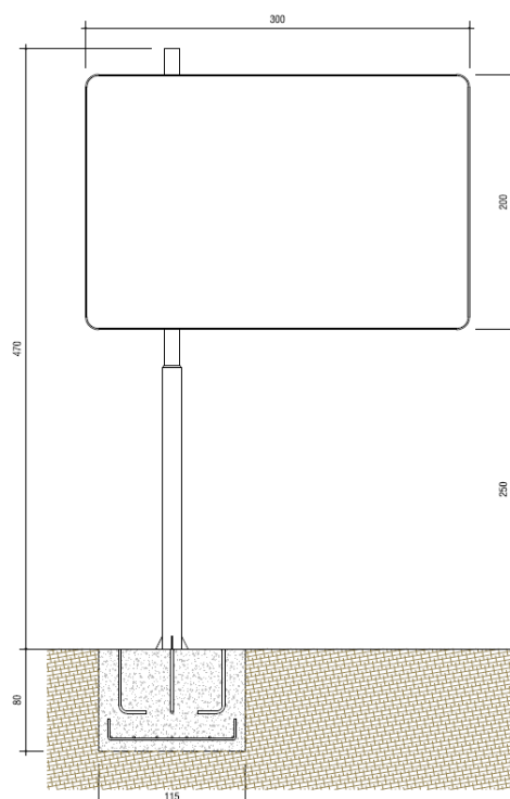
Dibuix alçat frontal
