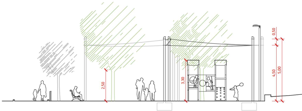
Vista sud de la proposta plantejada a la zona de jocs infantils de la Plaça Lluís Companys
