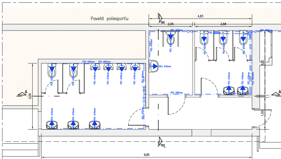
PLANTA BAIXA (SERVEIS HIGIÈNCIS) Esc. 1:50
