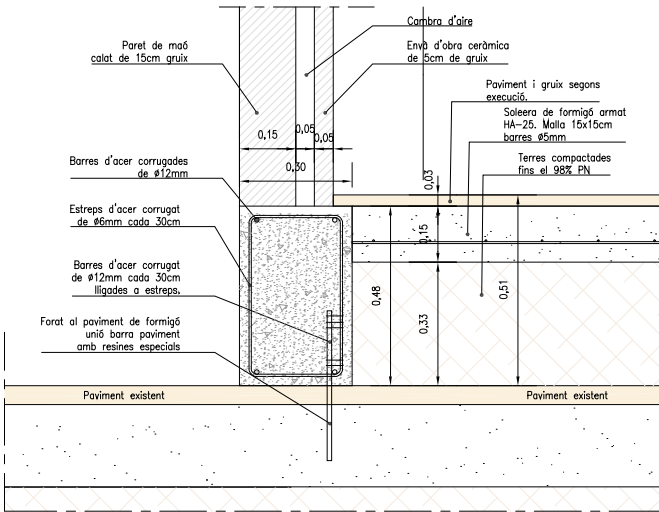
SECCIÓ C-C Esc. 1:50
