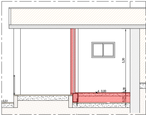
SECCIÓ C-C Esc. 1:50
