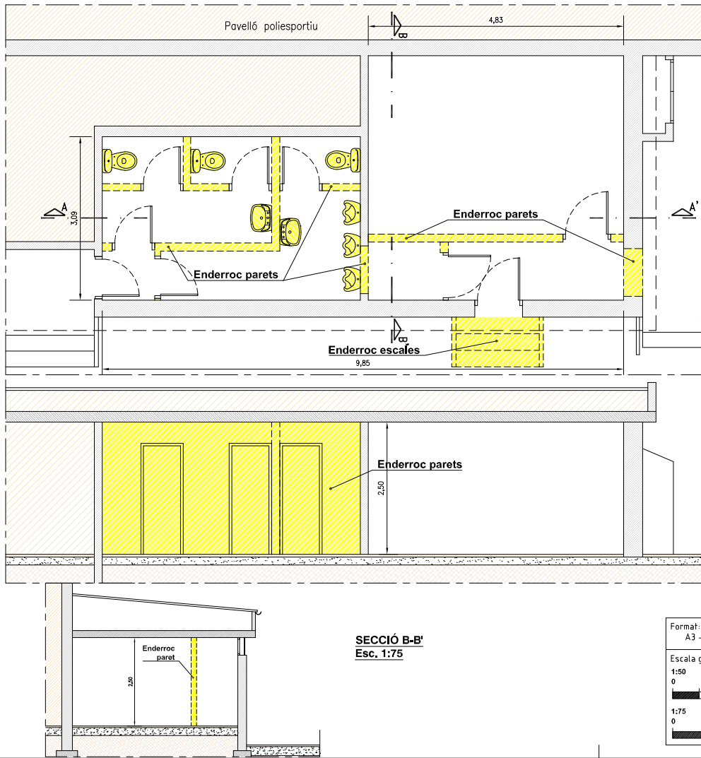
PLANTA BAIXA (SERVEIS HIGIÈNICS) Esc. 1:50
