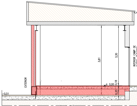
SECCIÓ A-A Esc. 1:50
