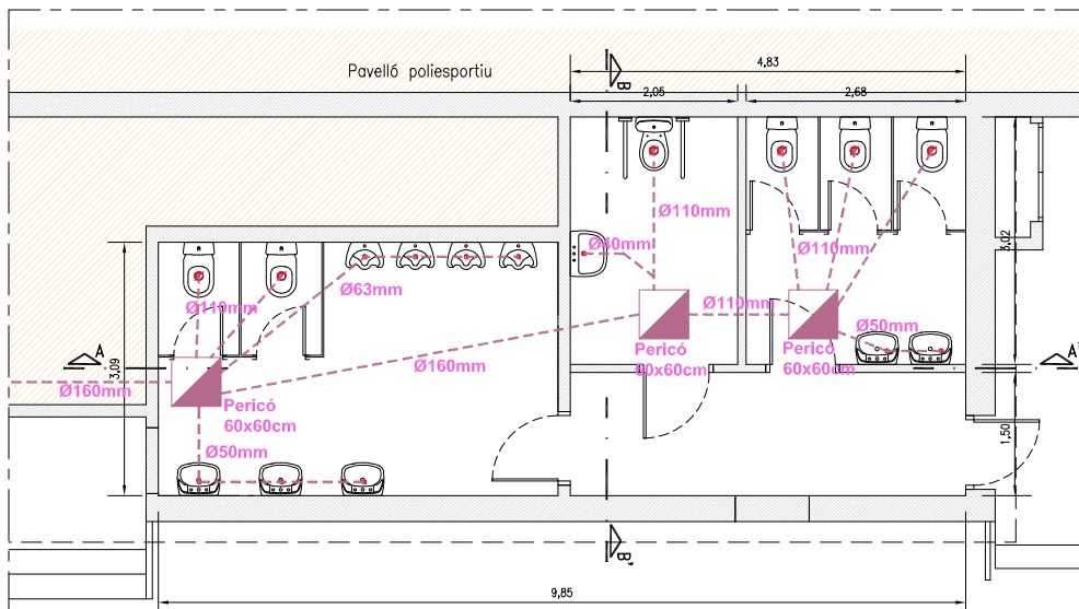
PLANTA BAIXA (SERVEIS HIGIÈNICS) Esc. 1:50
