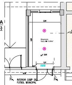
PLANTA BAIXA (MAGATZEMS) Esc. 1:100
