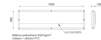
18. MATALÀS 3D
