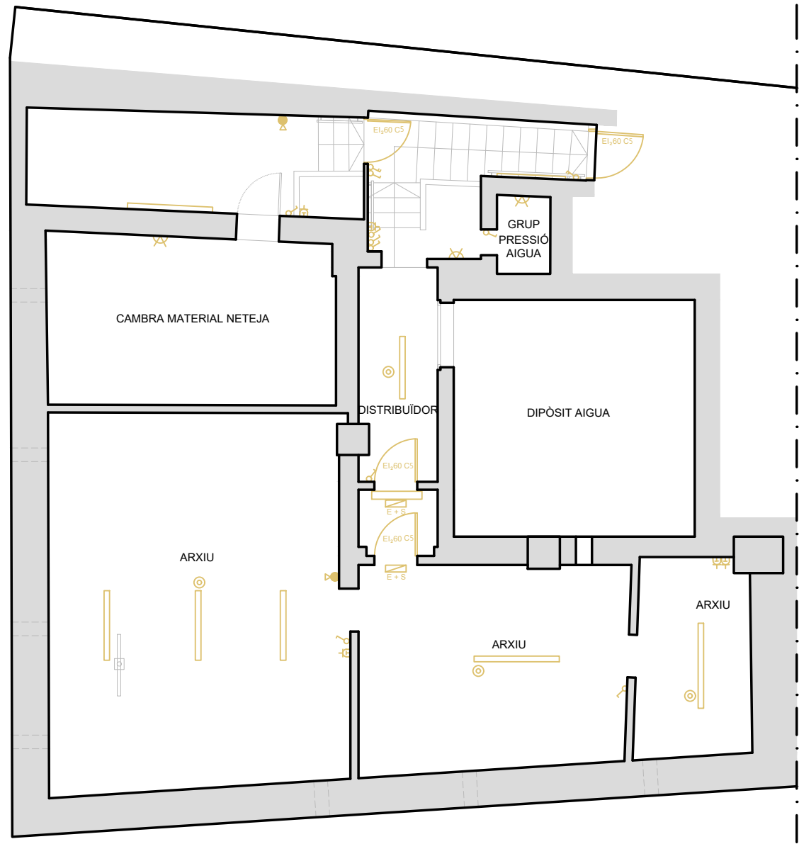
PLANTA SOTERRANI . PROPOSTA ESC:1/50
