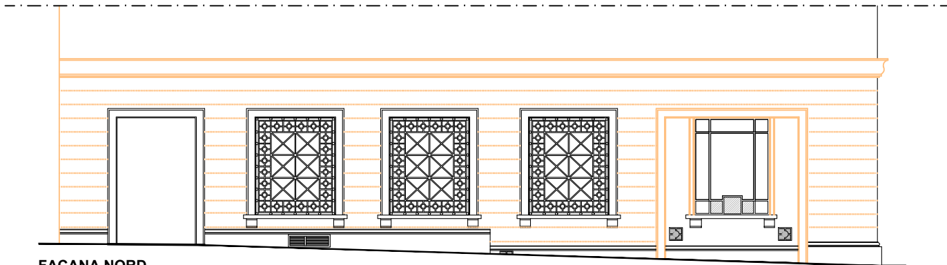
FAÇANA NORD . C/ AGODERS ESC:1/100
