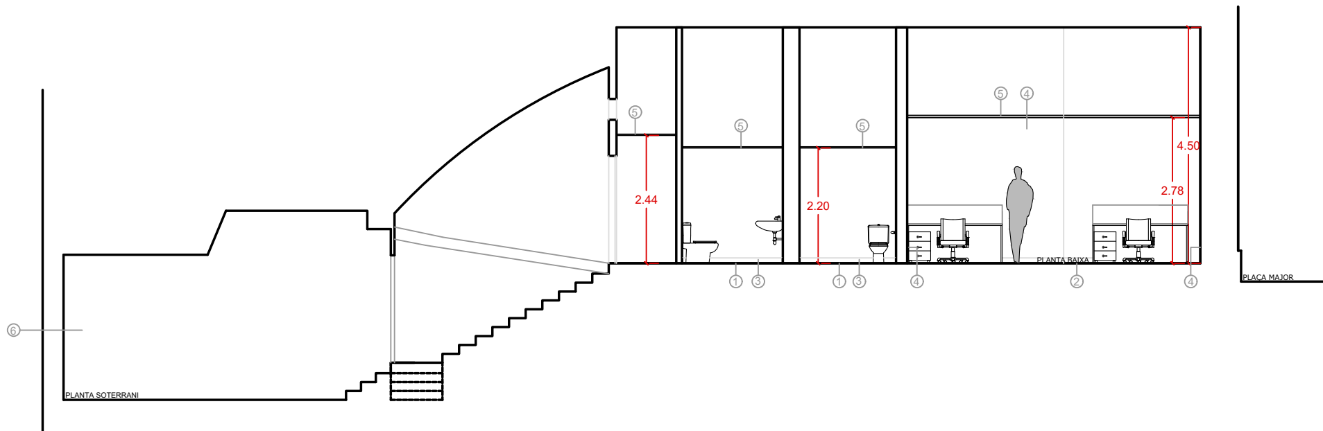
SECCIÓ -S3-
