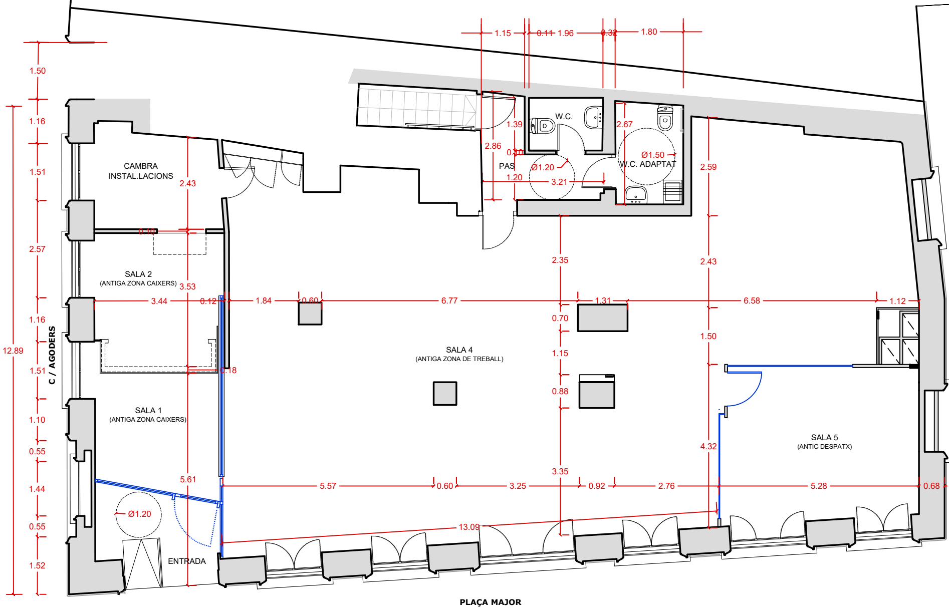
PLANTA BAIXA . ESTAT ACTUAL ESC:1/50
