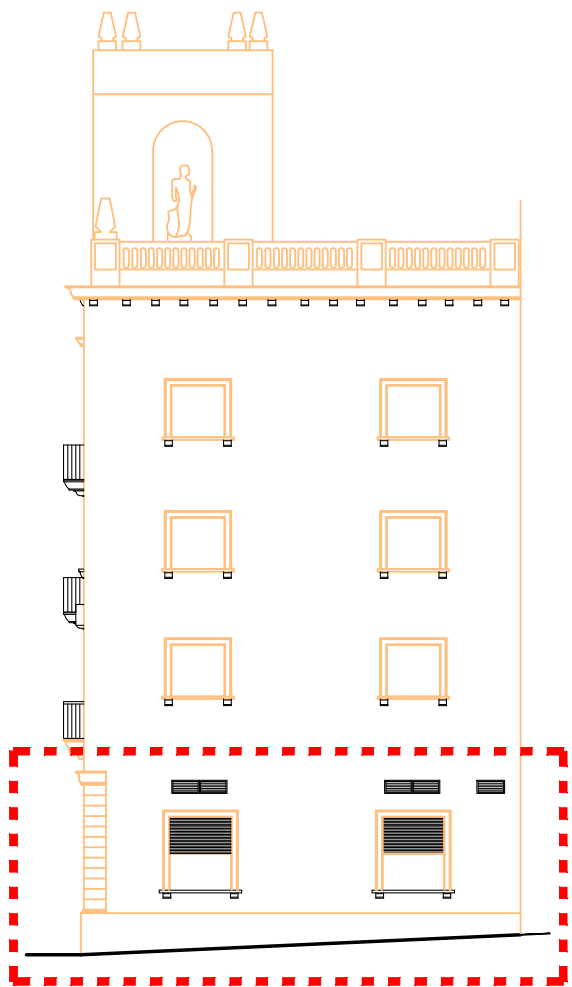
FAÇANA SUD . ESC:1/200
