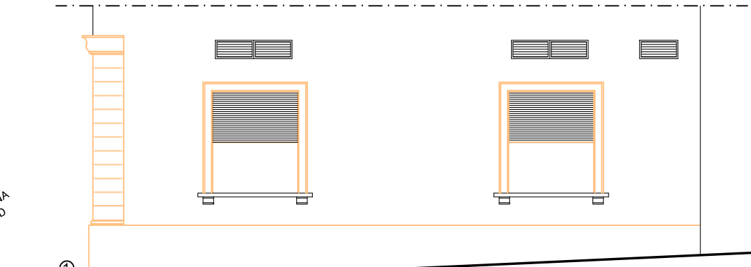
FAÇANA SUD . ESC:1/100
