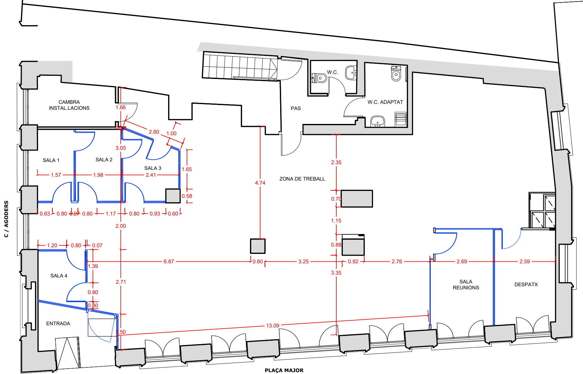
PLANTA BAIXA . PROPOSTA ESC:1/50
