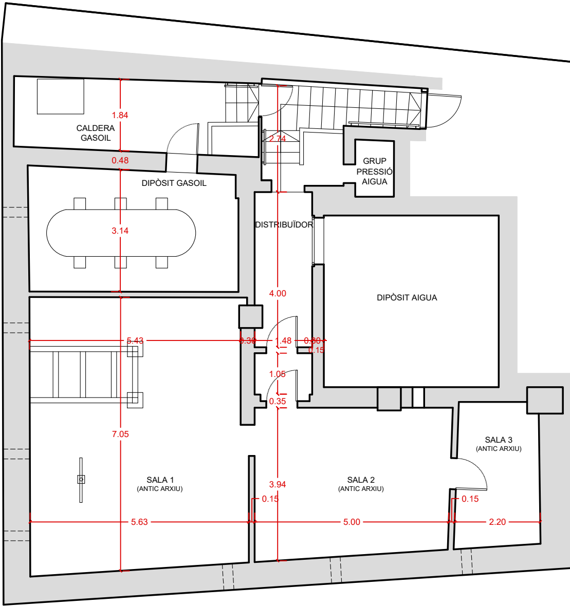
PLANTA SOTERRANI . ESTAT ACTUAL ESC:1/50
