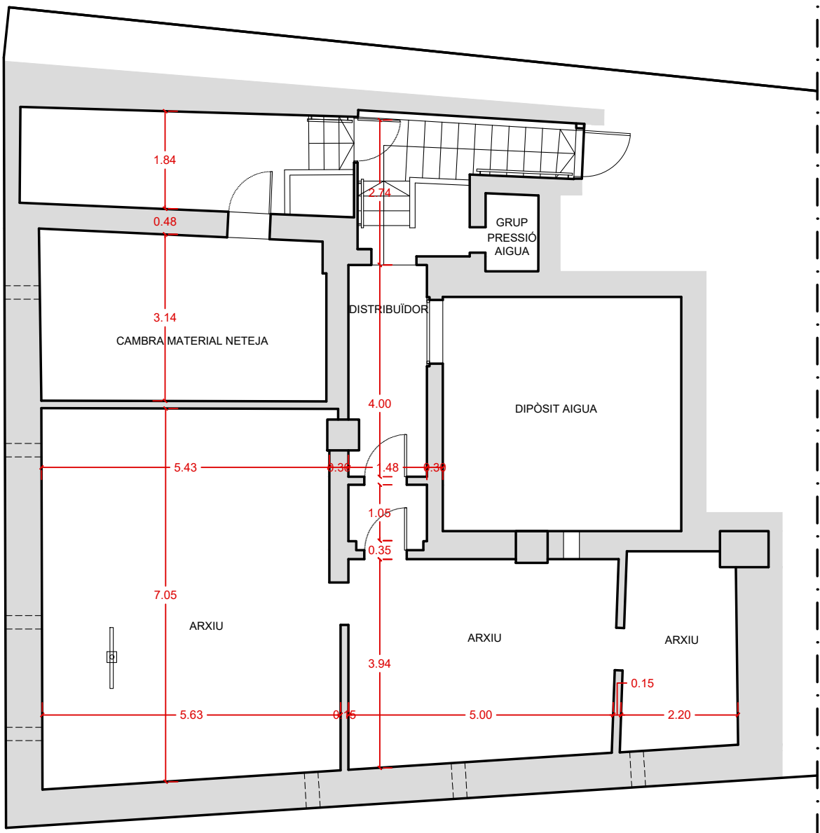
PLANTA SOTERRANI . PROPOSTA ESC:1/50
