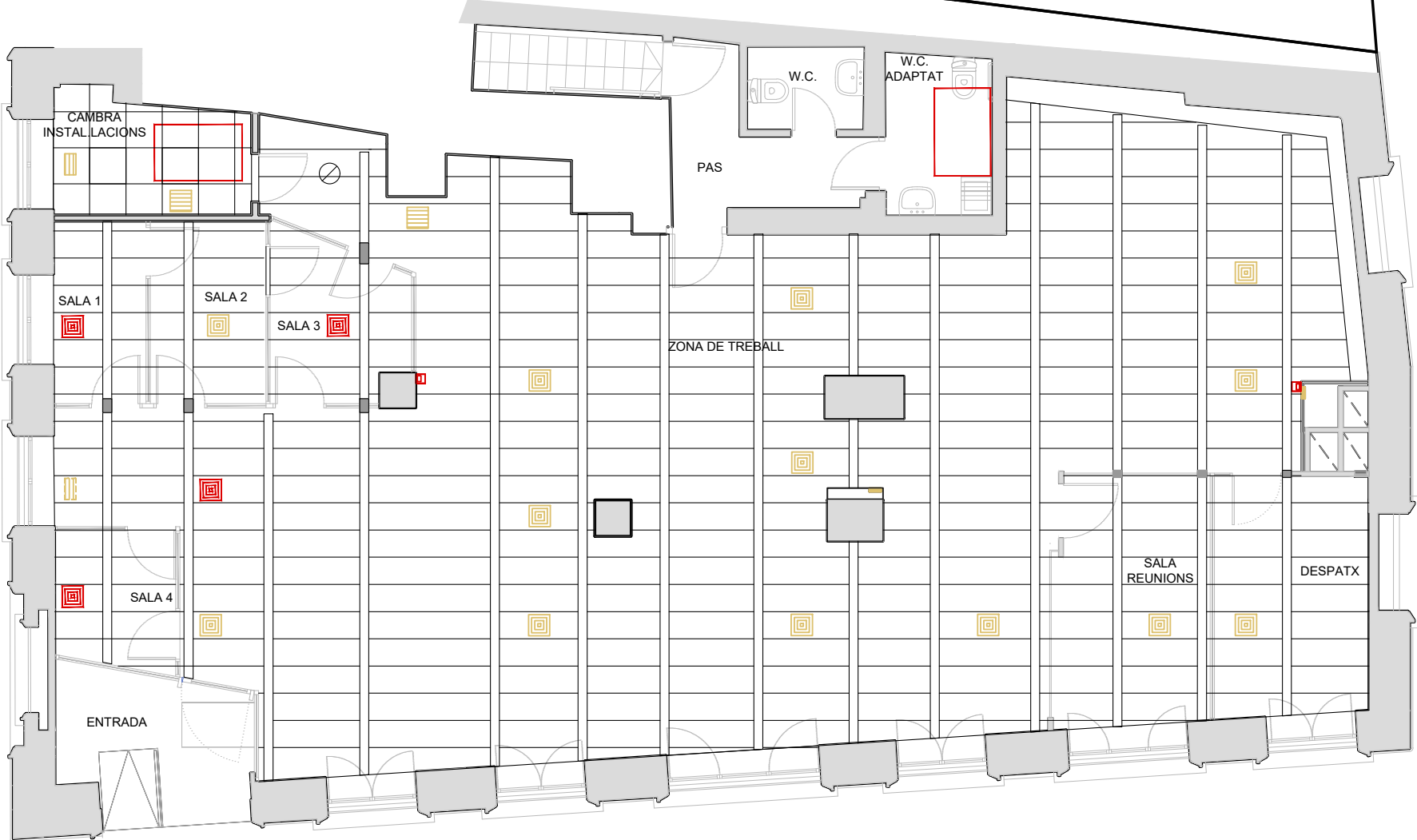
PLANTA BAIXA . PROPOSTA ESC:1/50
