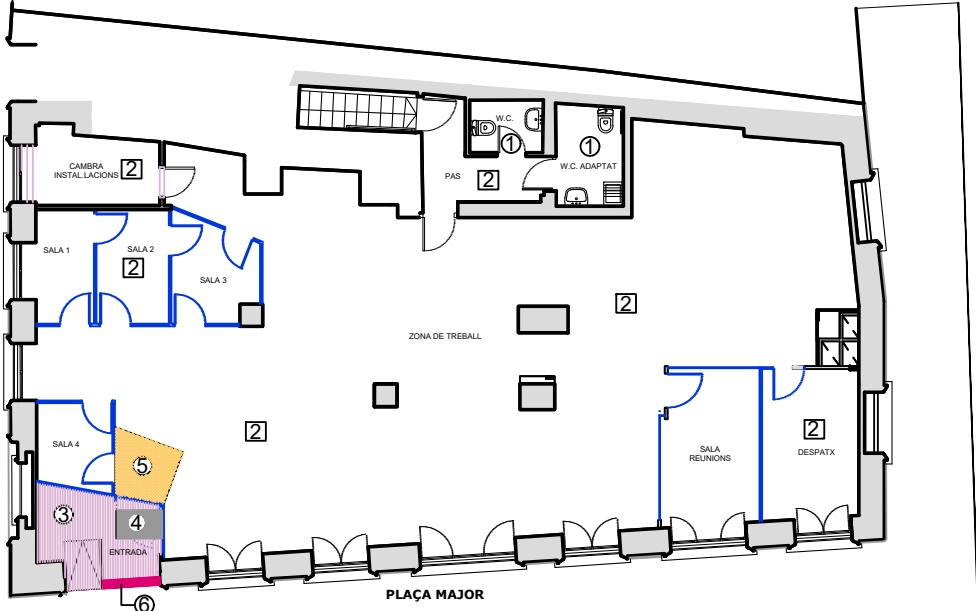
PLANTA PAVIMENTS. PROPOSTA ESC:1/100
