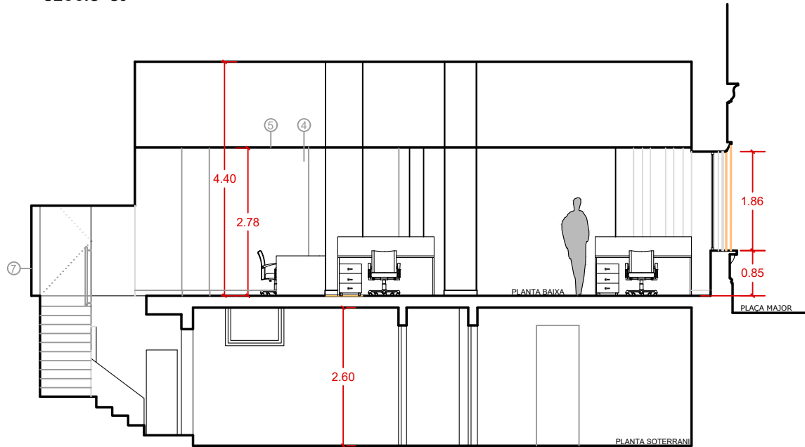
SECCIÓ -S4-
