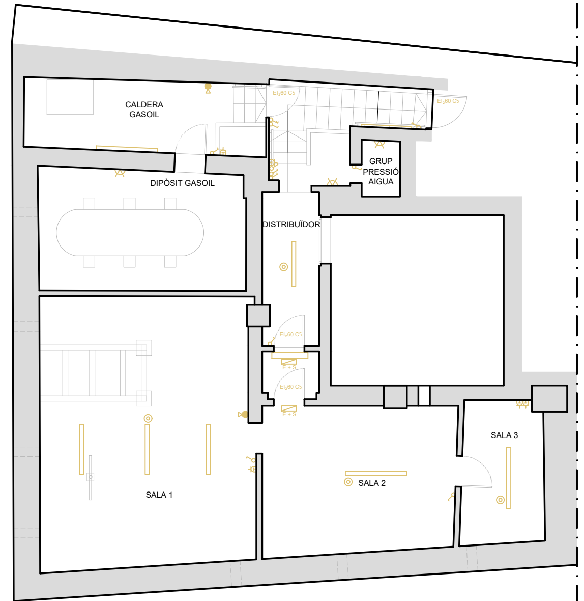
PLANTA SOTERRANI . ESTAT ACTUAL ESC:1/50
