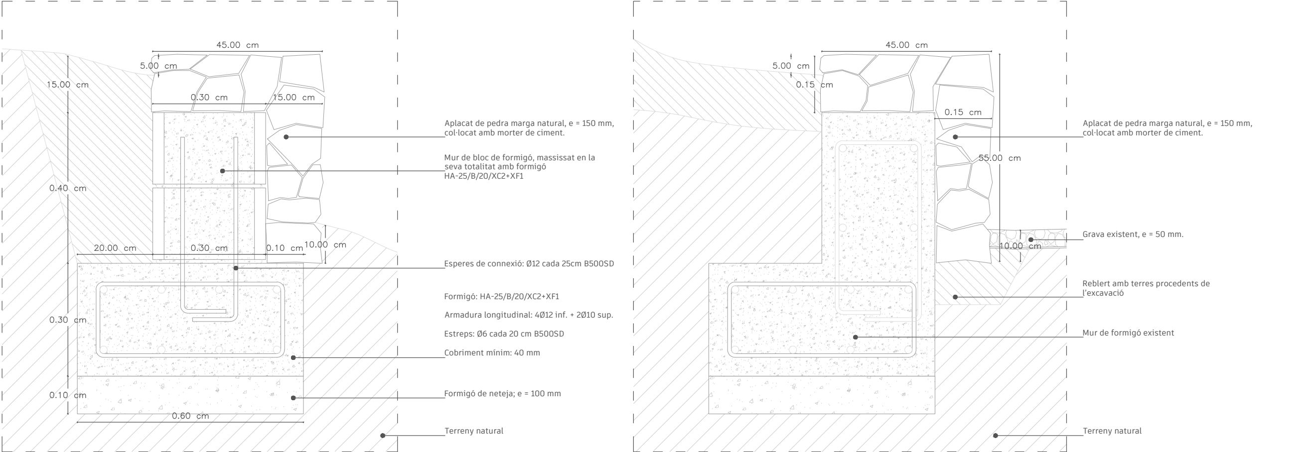
Detall del nou muret de bloc, e: 1_10
