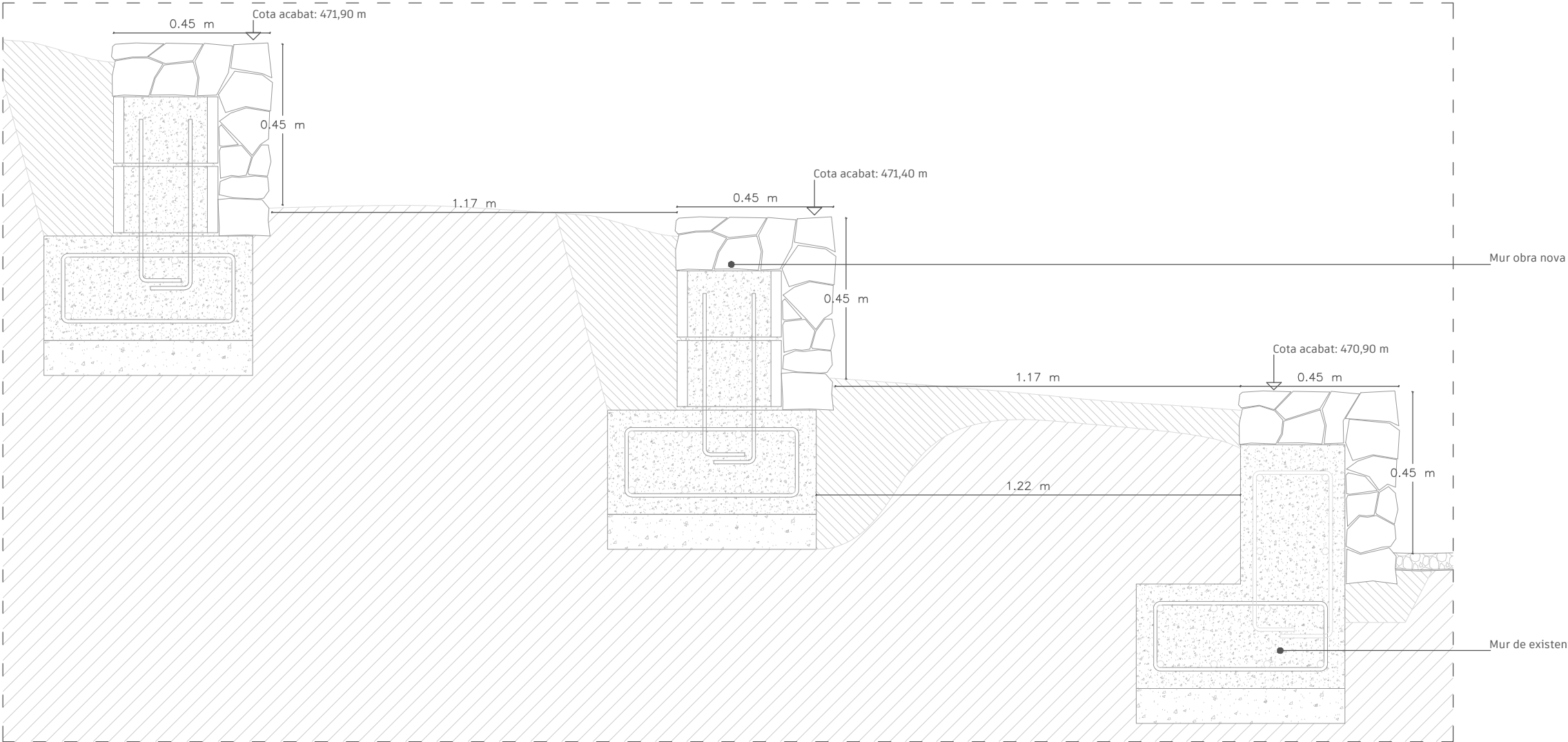
Secció A-A', e: 1_15
