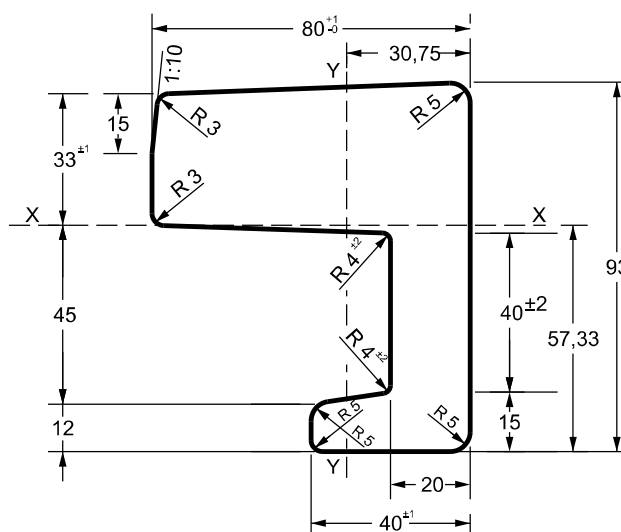
PERFIL DE CONTRACARRIL 33C1
