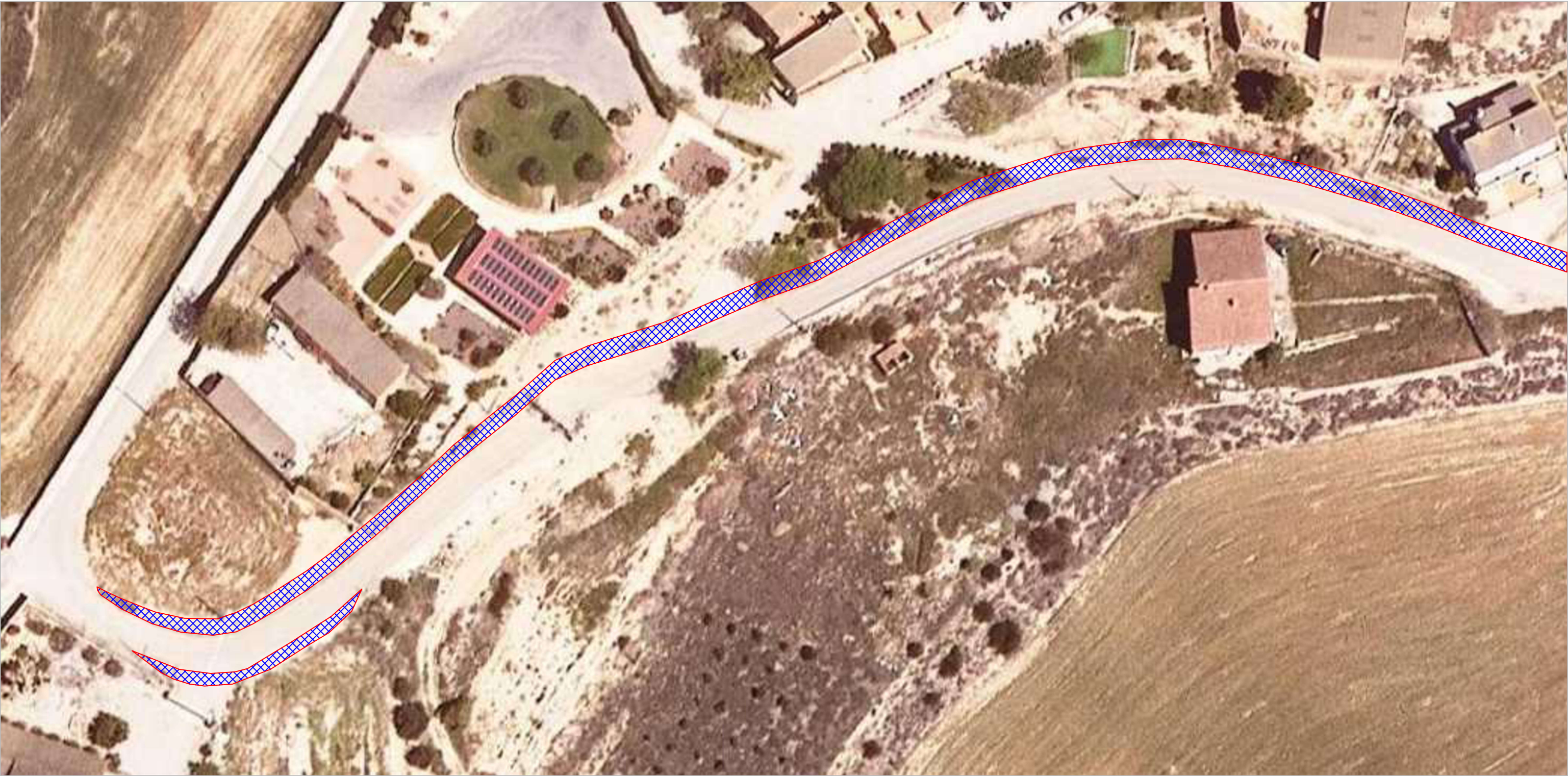
EIXAMPLAMENT DEL VIAL D'ACCÉS AL NUCLI DE LA MORANA AMB PAVIMENT DE FORMIGÓ, LONGITUD TOTAL 531 m LINIALS, AMPLADA MITJA 1,25 m, GRUIX PAVIMENT DE FORMIGÓ 17 cm
