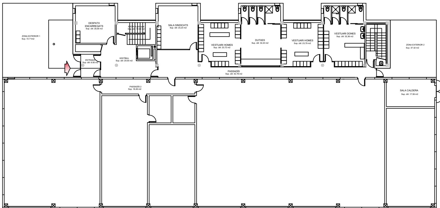
Edifici Neteja Viària PLANTA BAIXA
