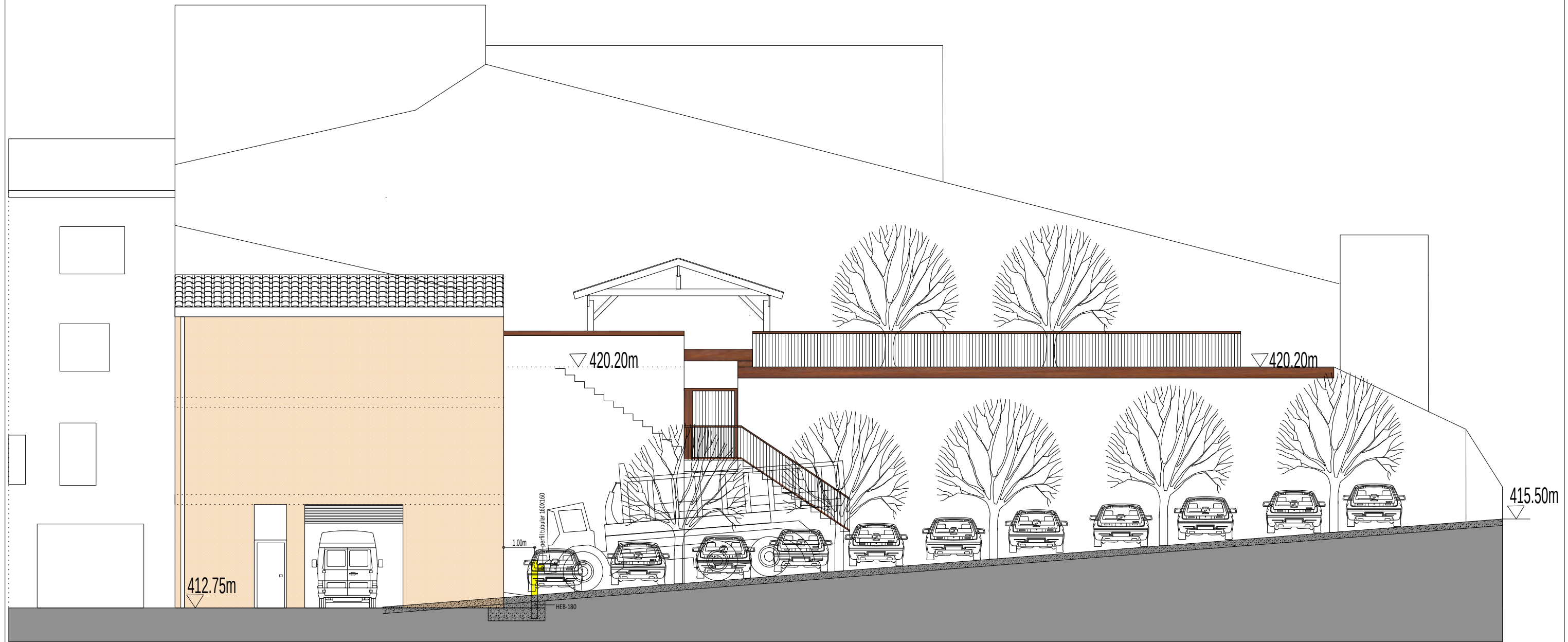
ALÇAT PER CARRER MORE
