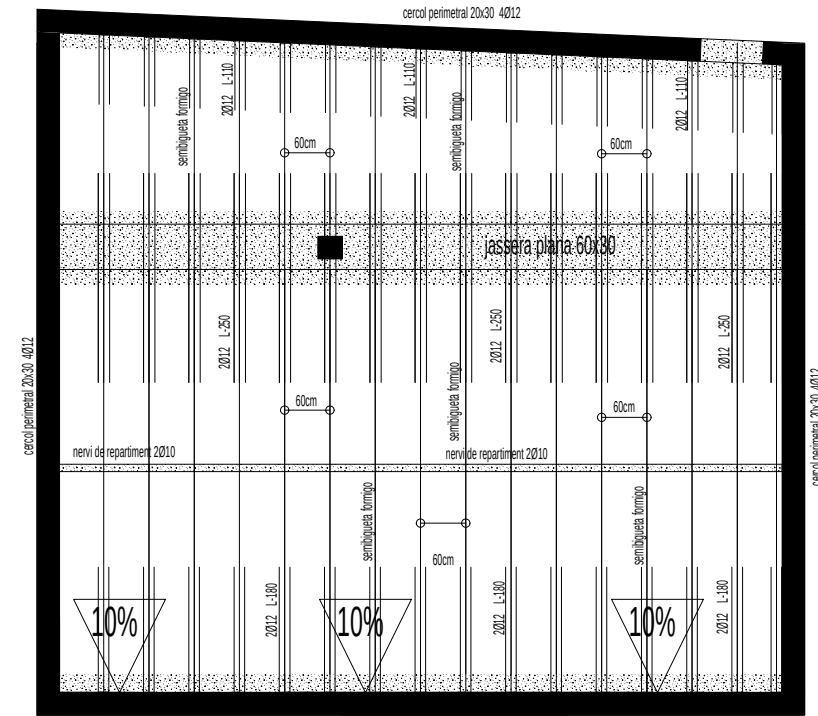
TEULADA
