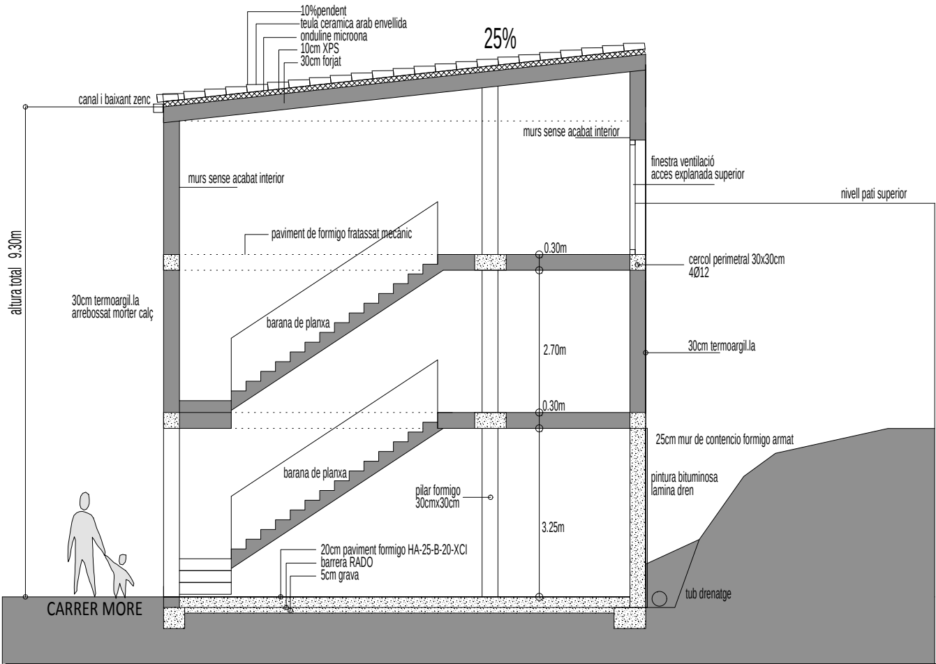
SECCIO TRANSVERSAL
