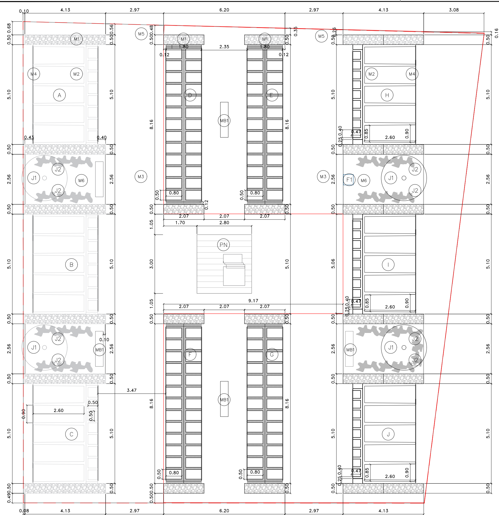
Planta cotes
