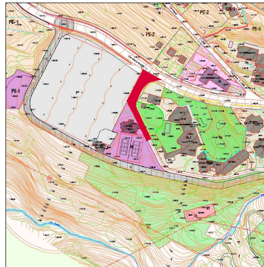
PLANEJAMENT URBANÍSTIC (Escala 1/2.500)
