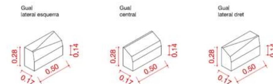
Figura 3: Definició de les tres tipologies de peça per a formació del qual sobre vorada.
