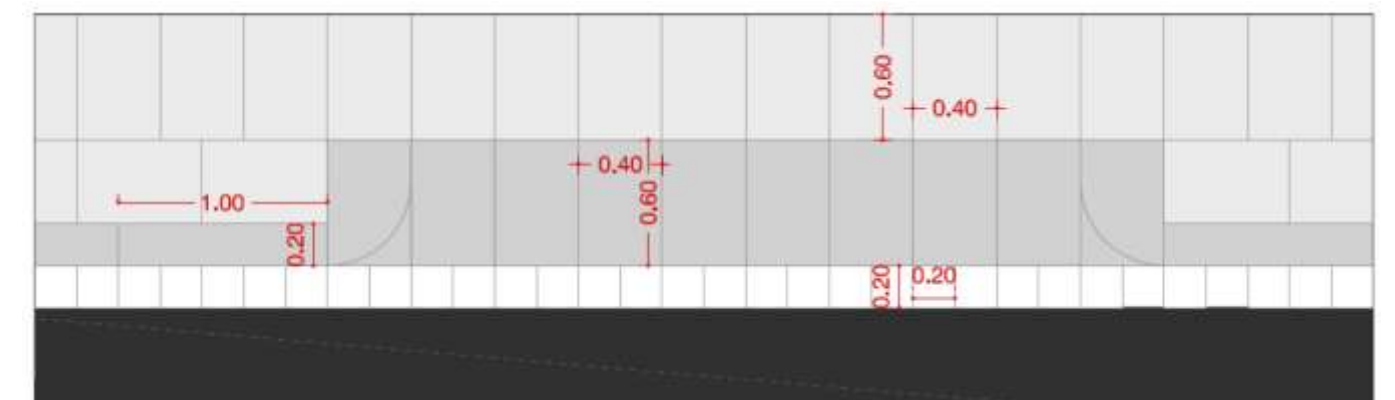
Figura 4: Esquema de qual tipus per els Carrers del Bisbe Morgades - Trams 2A i 2B.
