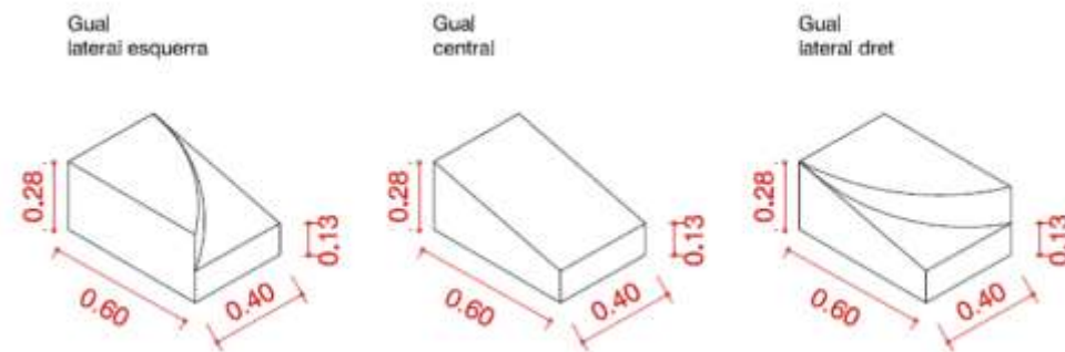
Figura 5: Definició de les tres tipologies de peça per a formació del gual tipus "V60".
