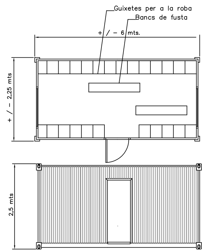
MÒDUL TIPUS DE VESTIDOR
