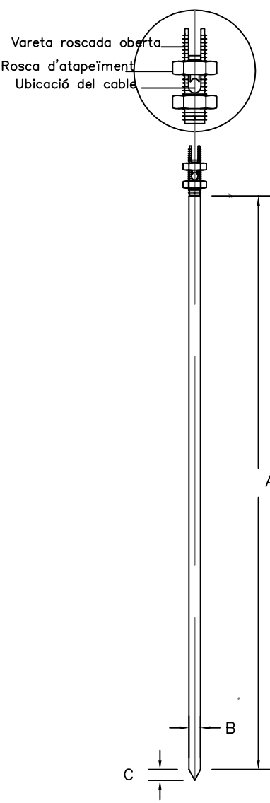
DETALL D'ANCORATGE DEL CABLE DE LA PICA
