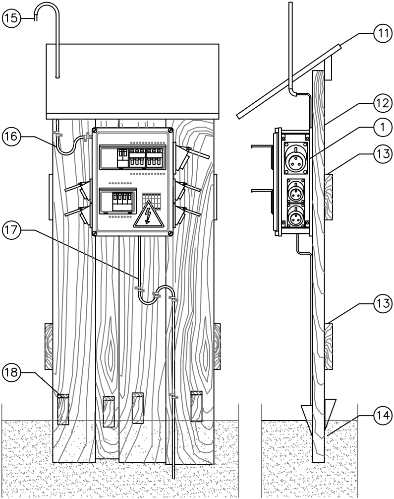
COL·LOCACIÓ TÍPICA DE QUADRE SECUNDARI ELÈCTRIC
