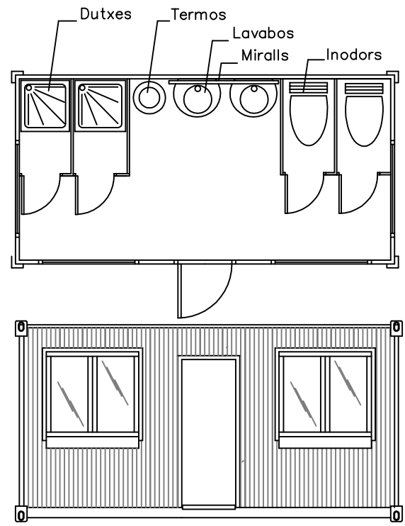
MÒDUL TIPUS DE LAVABO
