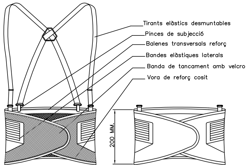
CINTURÓ ANTI-LUMBÀLGIA/ MOD. D'ACRÍLIC VELCRO
