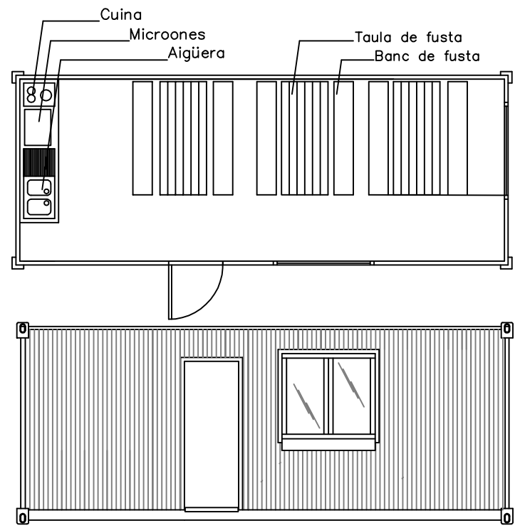
MÒDUL TIPUS DE MENJADORS
