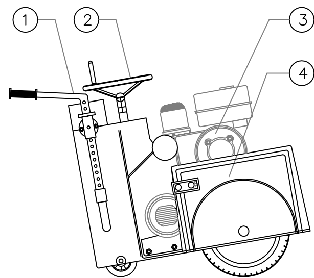
SERRA PER A PAVIMENTS (B)
