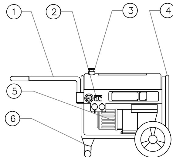
GRUP ELECTRÒGEN (C)
