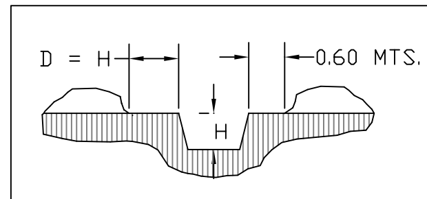
DISTÀNCIES DE SEGURETAT A LES RASES
