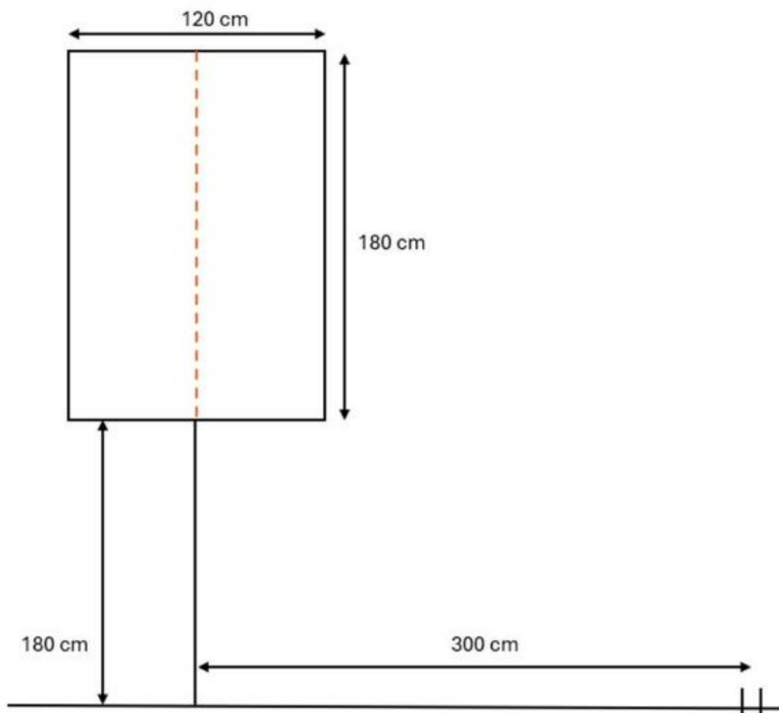
Fig. 4: Señal carretera N-230. Croquis de las medidas de los carteles y de las distancias de la señal con la vía de comunicación.
