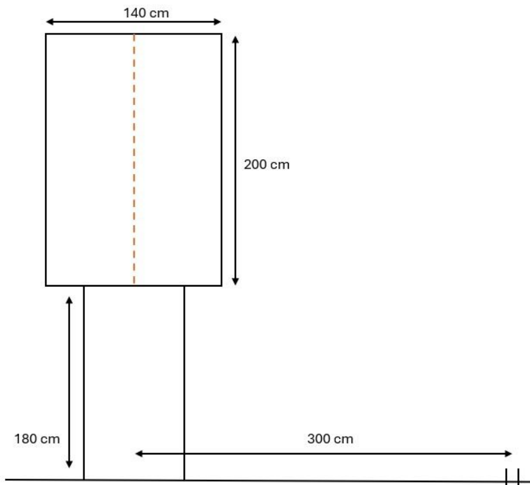
Fig. 6: Panell carretera C-28. Croquis de las medidas de los carteles y de las distancias de la señal con la vía de comunicación.
