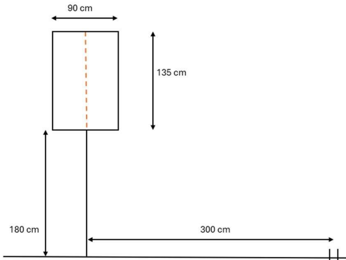
Fig. 5: Señal carretera N-141. Croquis de las medidas de los carteles y de las distancias de la señal con la vía de comunicación.
