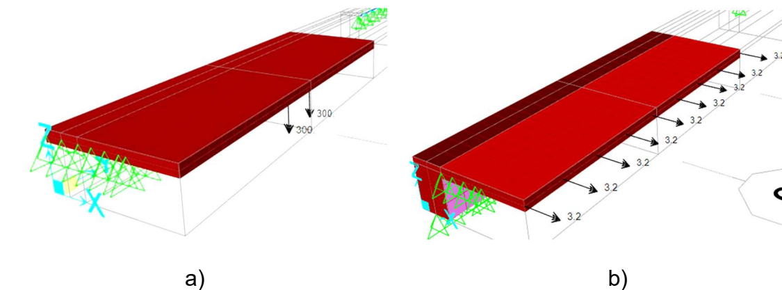
Il·lustració 8. a) Càrregues aplicades del vehicle pesant excèntric 30T, Sap 2000 y b) Càrregues de baranes.
