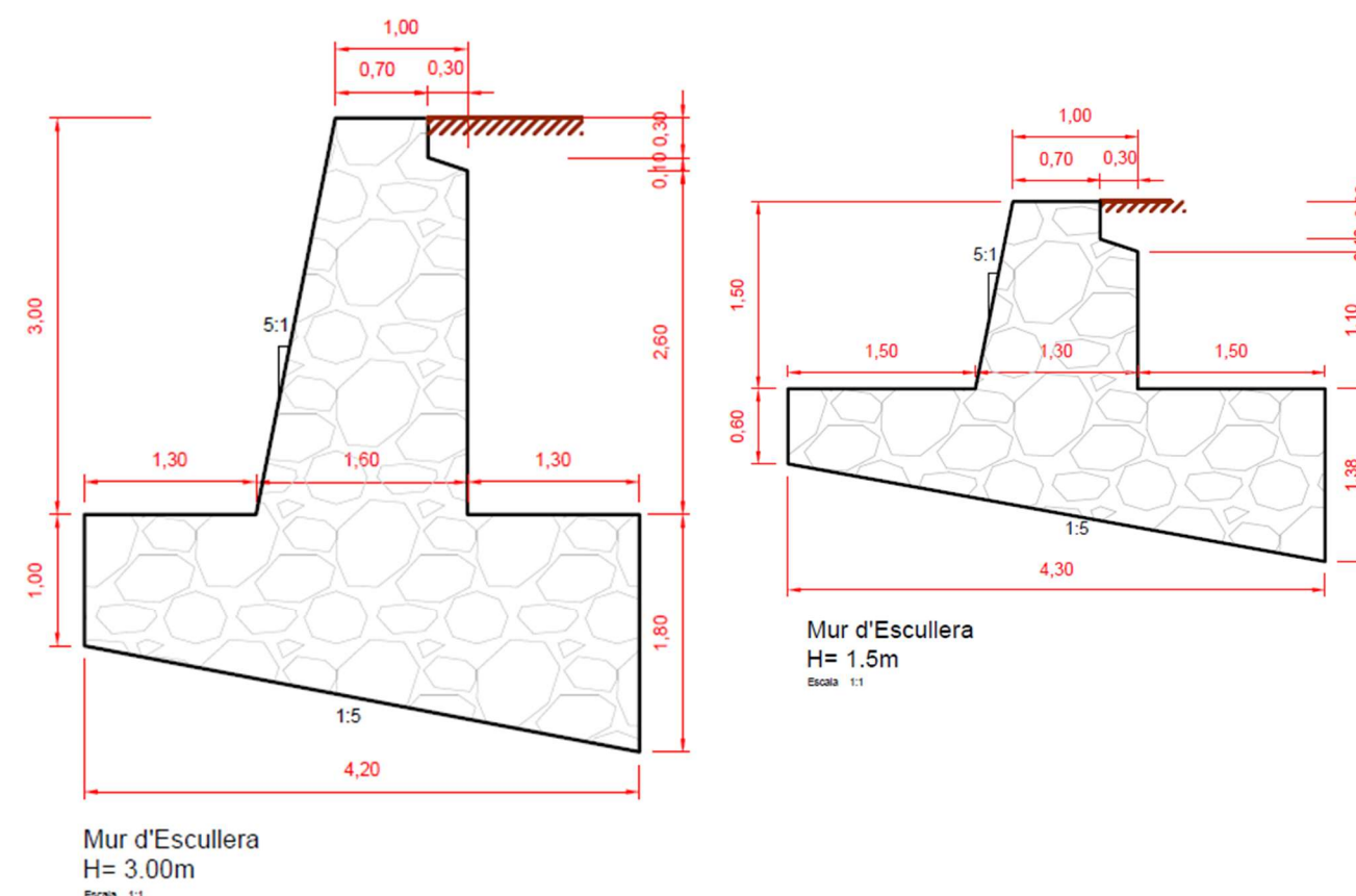
Il·lustració 10. Mur d'escullera per a un H=3,0m i H=1,5m
