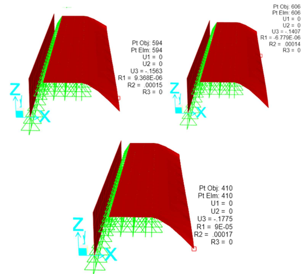
Il·lustració 12. Deflexions i deformacions seccionals en (mm), Sap 2000.
