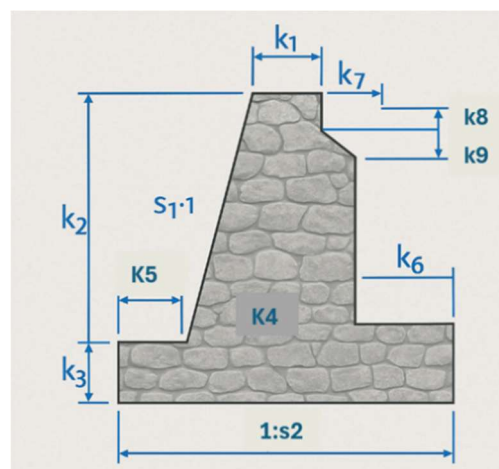
Il·lustració 9. Variables Geomètriques del mur d'escullera
