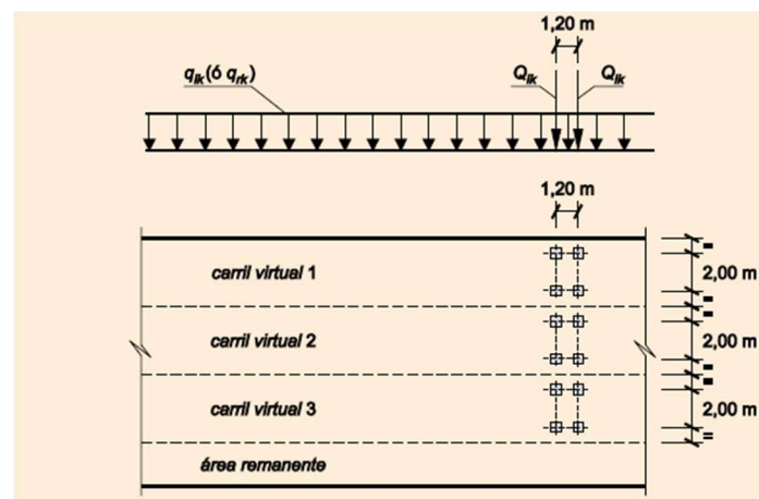
Il·lustració 6. Carrils virtuals i distàncies entre eixos de les rodes vehiculassis.
