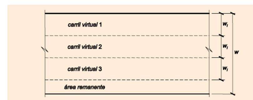
Il·lustració 4. Carrils virtuals d'acord amb el IAP-11.
