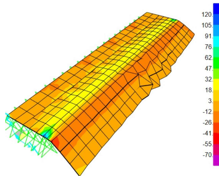
Il·lustració 13. Diagrama de tallants X-X en la secció en (KN). Sap 2000.
