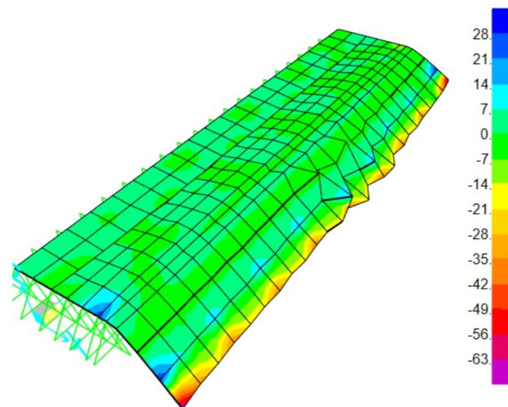
Il·lustració 14. Diagrama de tallants Y-Y en la secció en (KN). Sap 2000.
