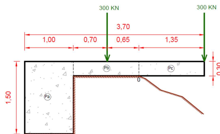
Il·lustració 11. Esquema d'anàlisi d'equilibri davant volteig
