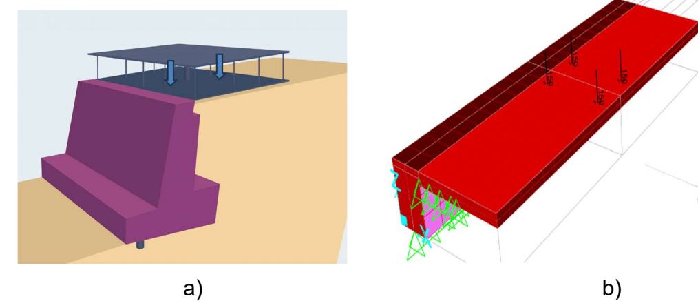
Il·lustració 7. Càrregues aplicades del vehicle pesant centric 60T, Sap 2000.
