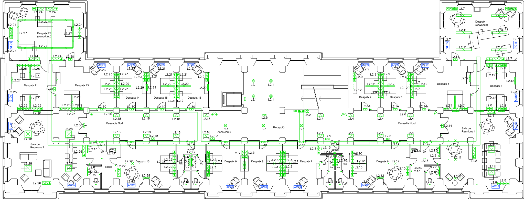
PLANTA PRIMERA
