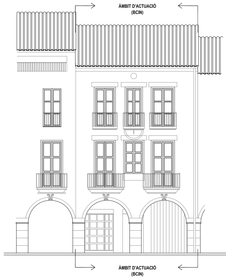
FAÇANA ESTAT ACTUAL PLAÇA GRAN Esc.: 1/150
