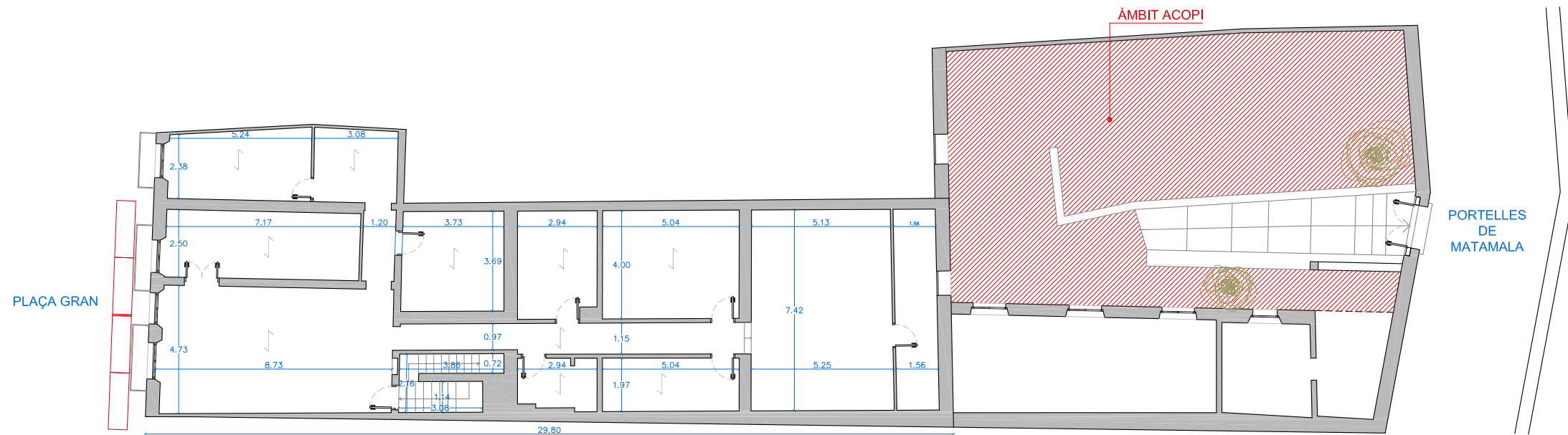
PLANTA PRIMER PIS ESTAT ACTUAL Esc.: 1/200
