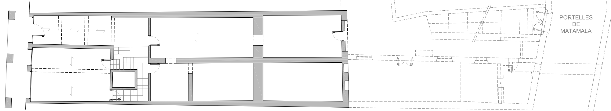
PLANTA BAIXA ESTAT ACTUAL PATI POSTERIOR C. PORTELLES Esc.: 1/200
