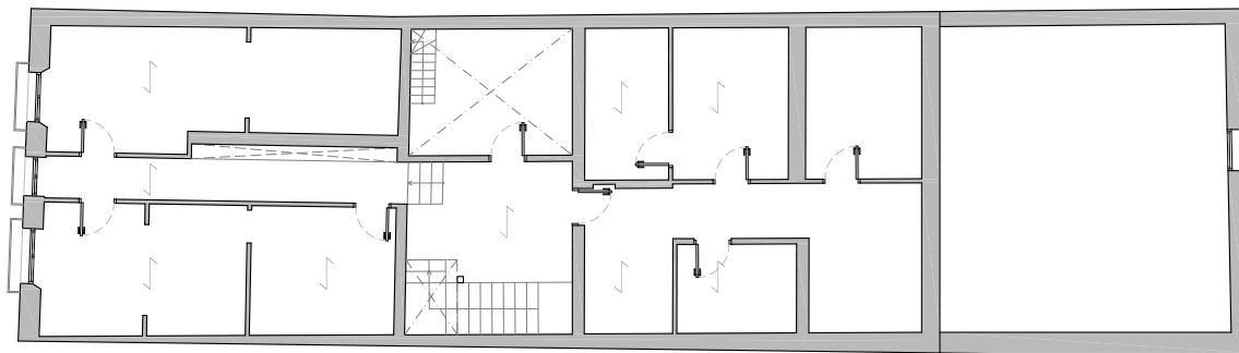
PLANTA SEGON PIS ESTAT ACTUAL Esc.: 1/200
