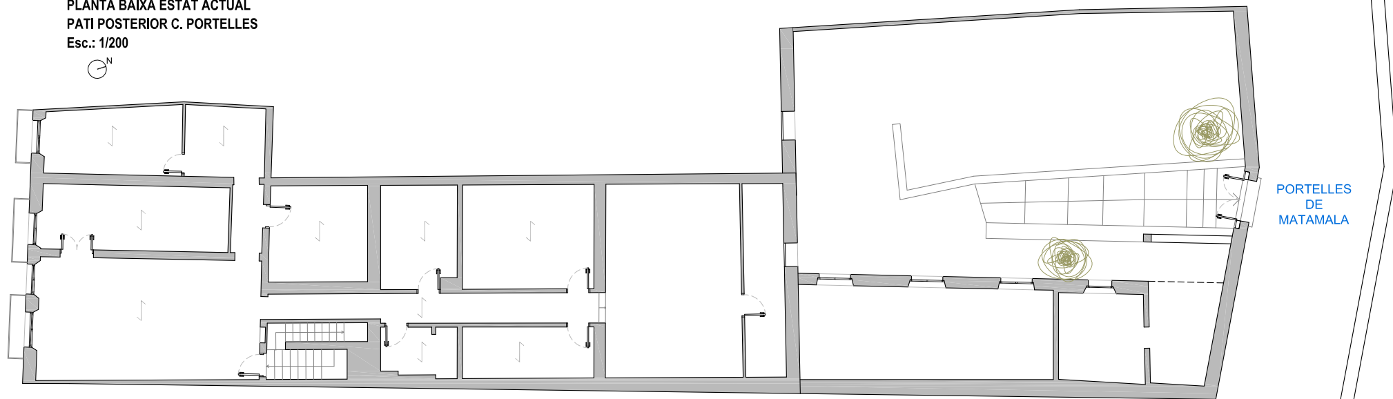
PLANTA PRIMER PIS ESTAT ACTUAL Esc.: 1/200
