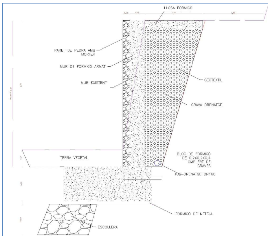
Il·lustració 3 Dimensions del mur projectat.
