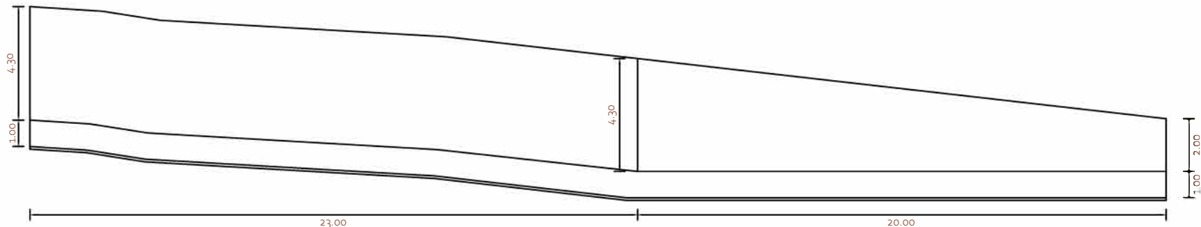
Tram de mur de 20 m d'alçada variable de 2 a 4.3m.
