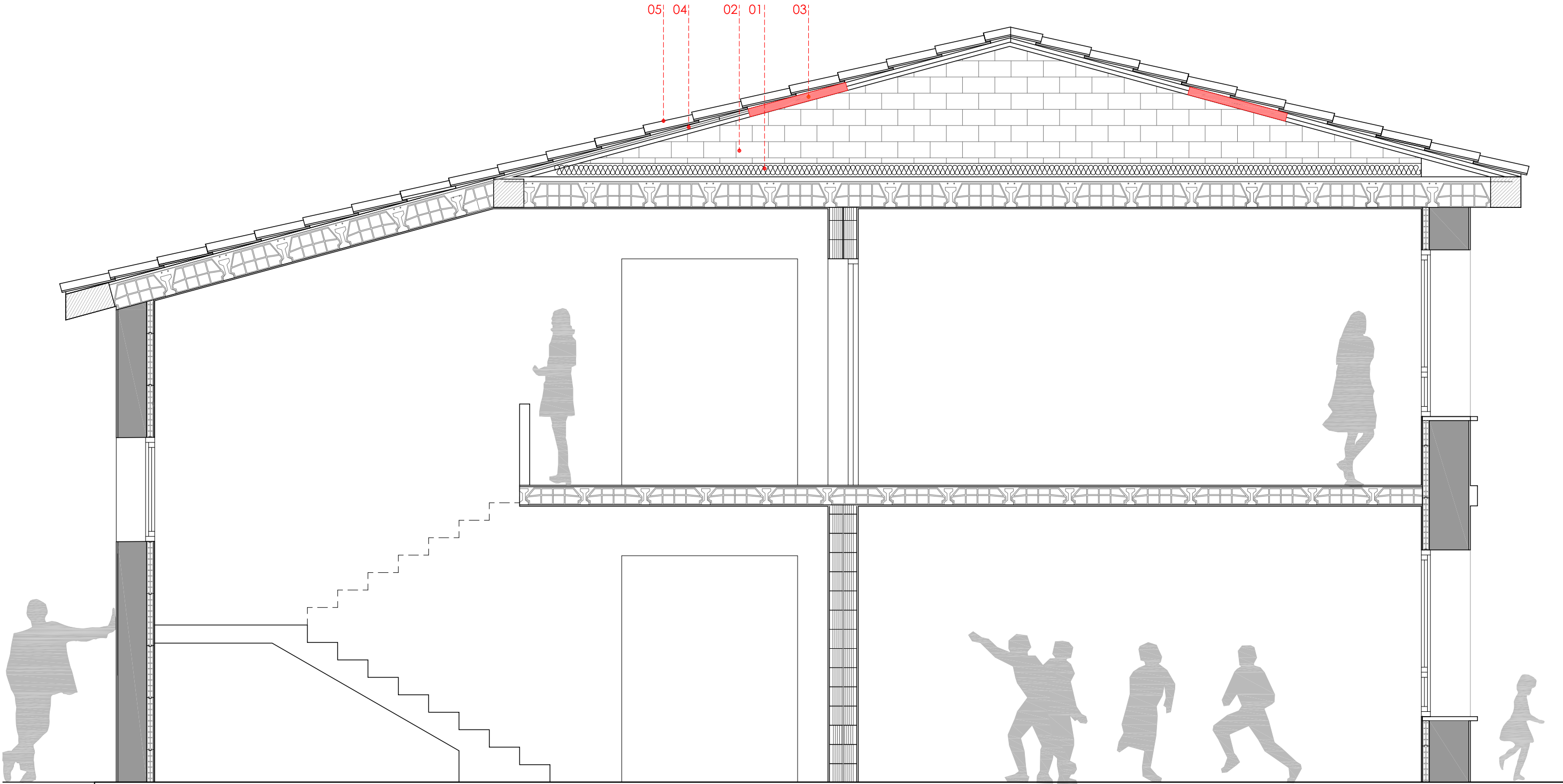
SECCIÓ TRANSVERSAL
