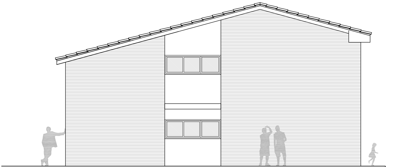
FAÇANA OEST
