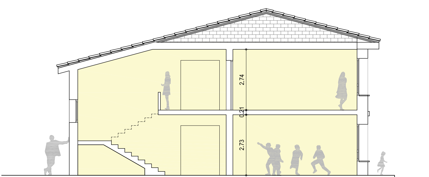
SECCIÓ TRANSVERSAL
